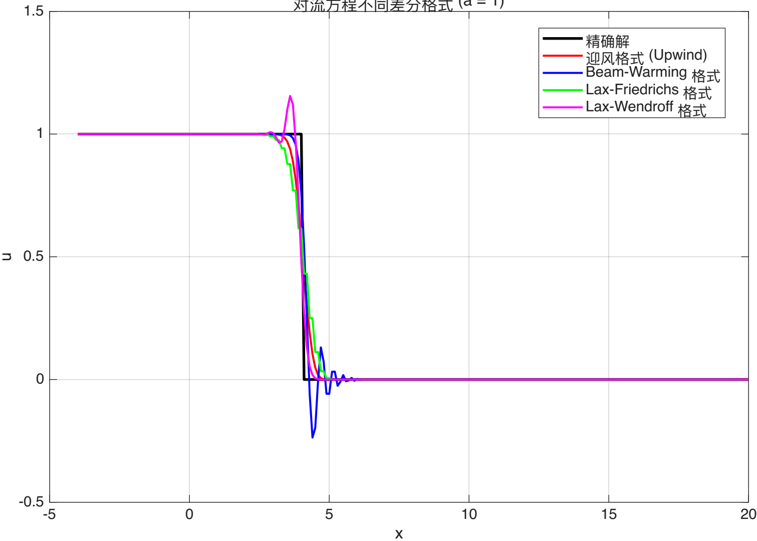
对流方程不同差分格式 (a = 1)
