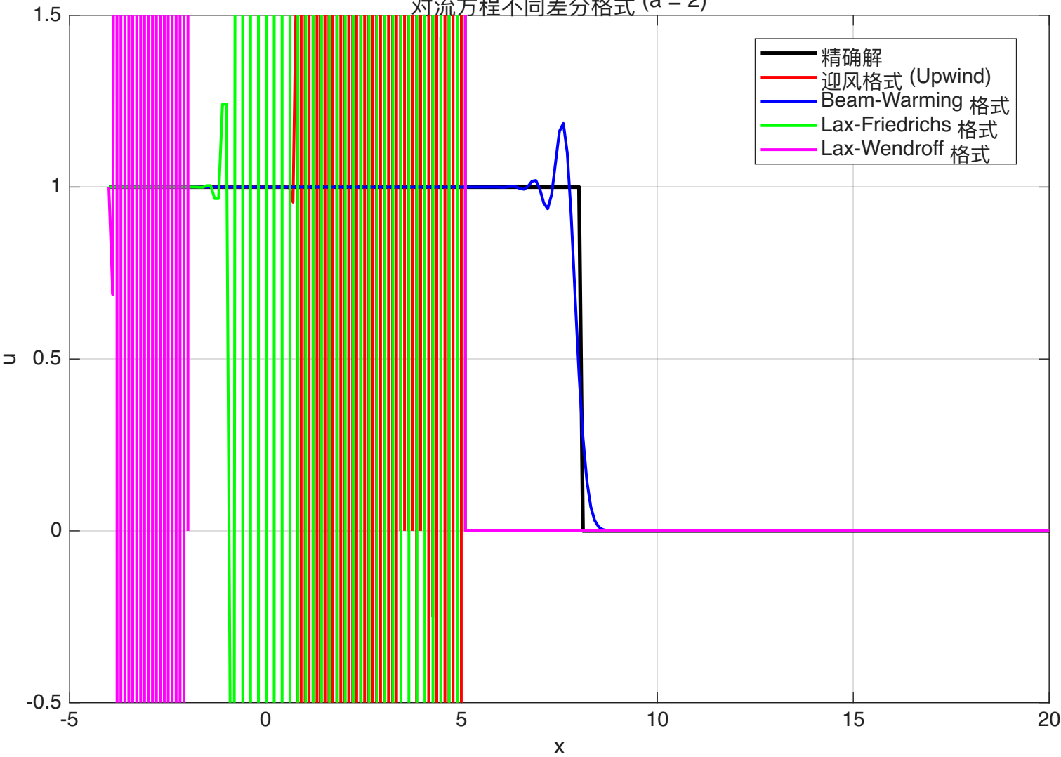
对流方程不同差分格式 (a = 2)
