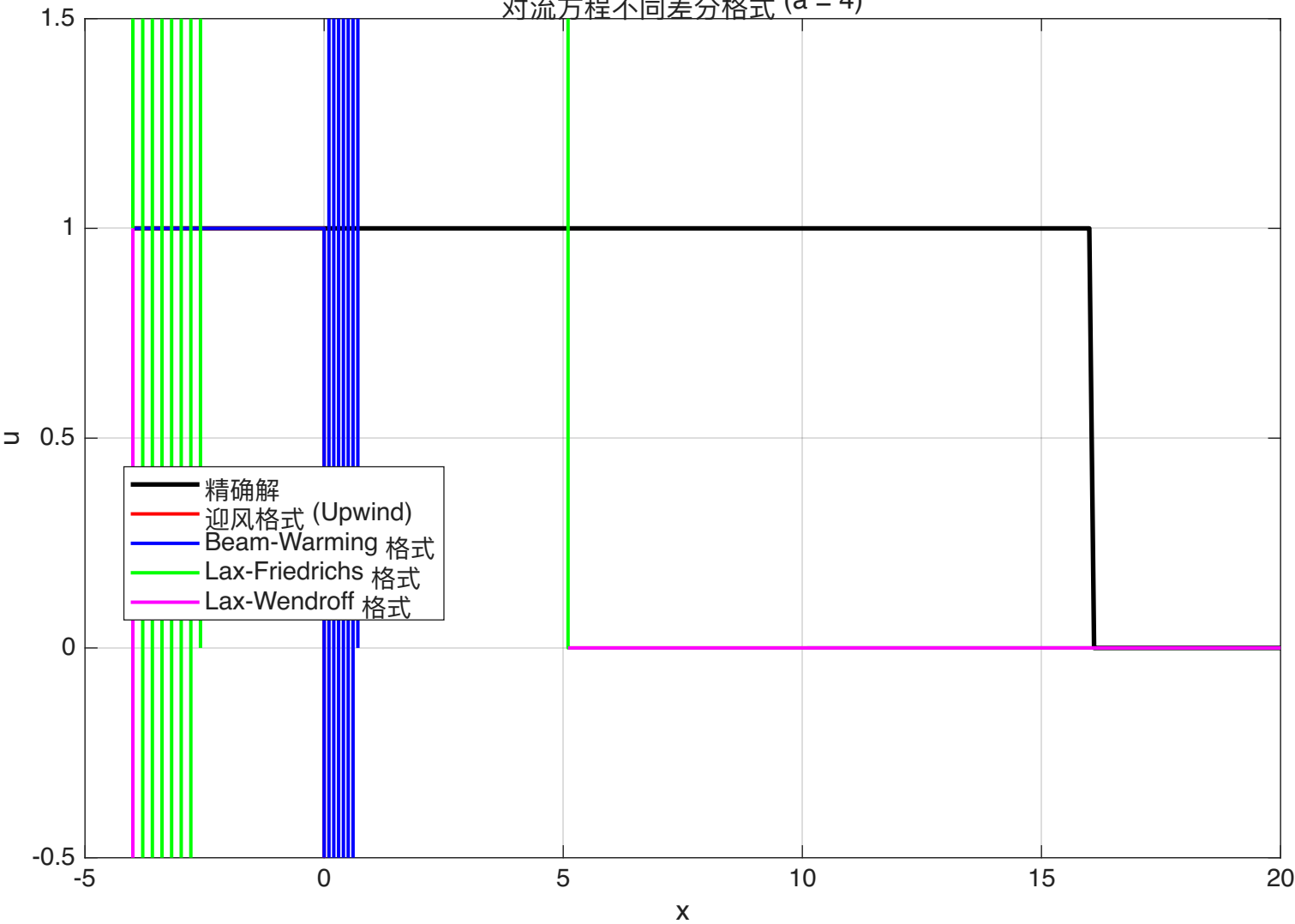
对流方程不同差分格式 (a = 4)
