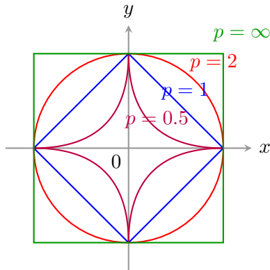
图 1.1: 不同 p 下的单位球
