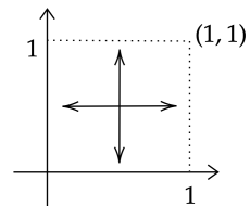
图 2.7: 二维环面
