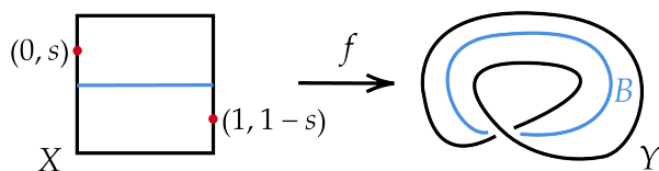
图 10.35: 莫比乌斯带的收缩
