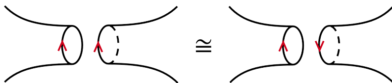
图 9.7: 粘合方式不影响连通和
