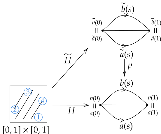
图 10.25: 同伦提升证明示意图
