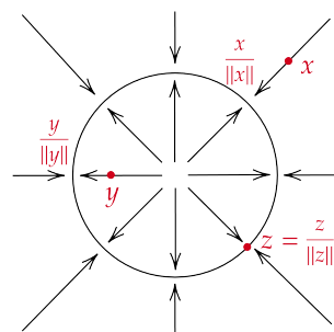
图 10.33: 到圆周上的形变收缩
