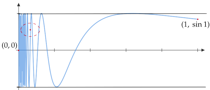
图 7.8: 拓扑学家正弦曲线
