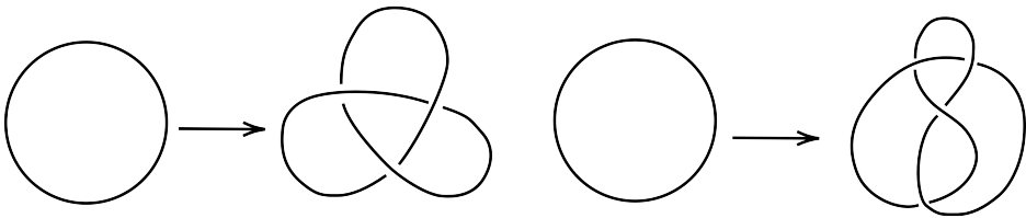
图 3.8: 纽结
