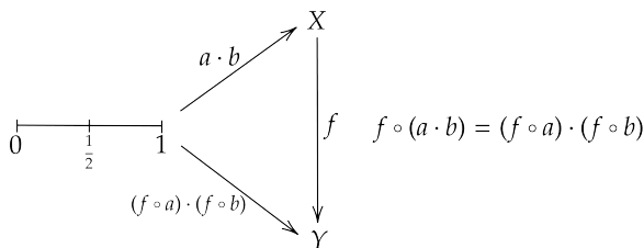
图 10.17: 证明图例
