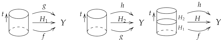
图 10.2: 同伦的传递性
