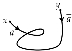
图 7.6: 逆道路
