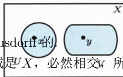
图 2.9: Hausdorff 性
