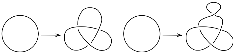
图 3.9: 同痕的纽结
