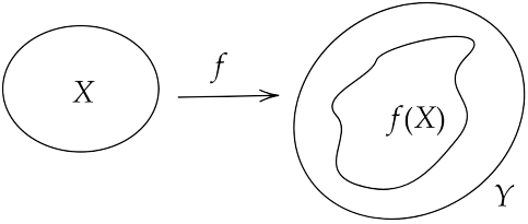
图 3.5: 嵌入
