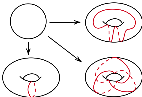
图 3.10: 圆环上的嵌入
