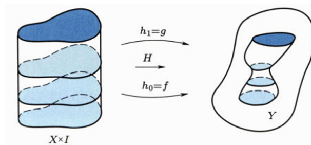
图 10.1: 同伦示意图
