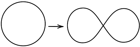
图 3.7: 非嵌入的映射
