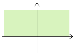
图 9.1: 上半平面 \mathbb{E}_+^2
