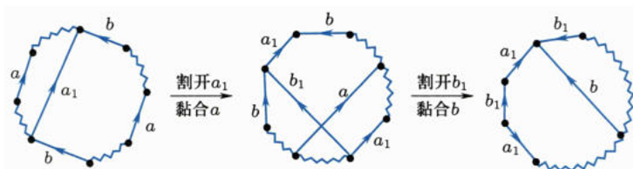
图 9.25: 对 a, b 分别作手术 B
