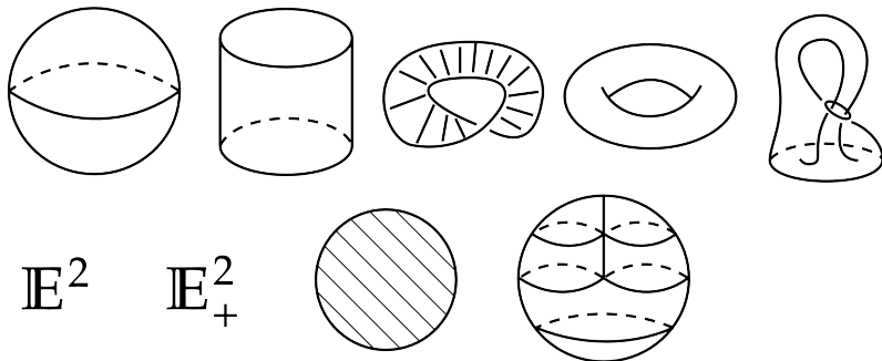
图 9.2: 曲面的例子
