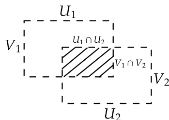
图 2.6: 乘积空间的拓扑基
