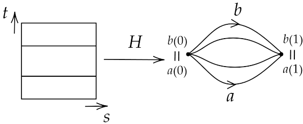
图 10.3: 道路同伦示意图 1
