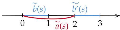
图 10.27: 道路连接
