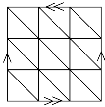
图 9.16: 克莱因瓶的三角剖分
