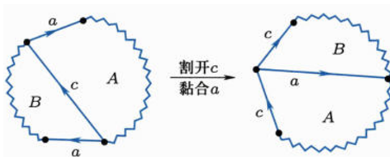
图 9.26: 用 (c, a) 作手术 B
