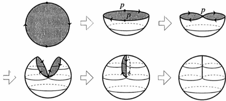
图 8.4: 射影平面的构造过程
