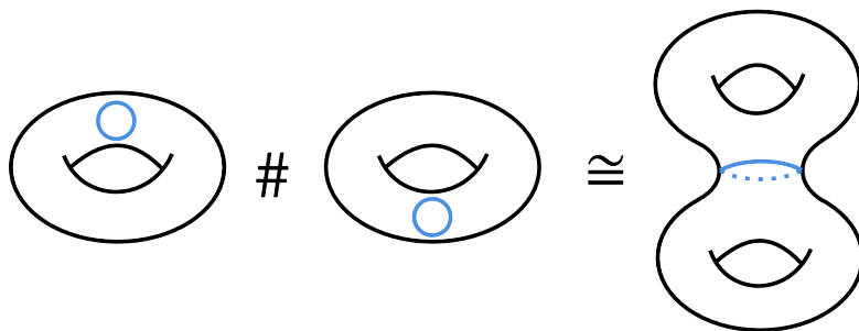
图 9.8: 移除开圆盘的位置不影响连通和
