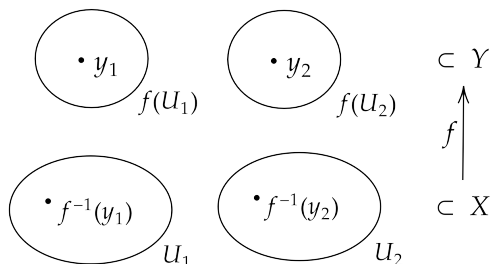
图 3.4: 同胚保持 Hausdorff 性质
