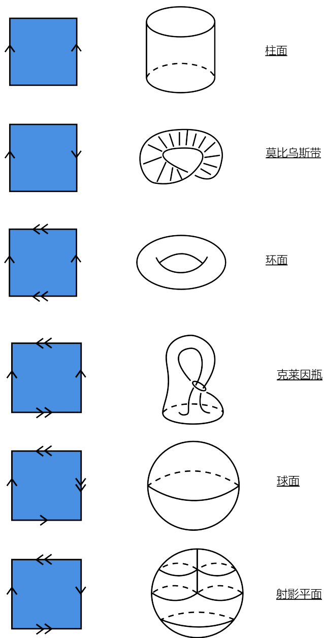
图 8.3: 正方形的商空间
