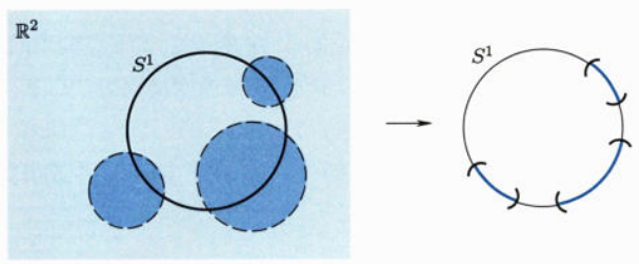
图 2.5: S^1 上的拓扑基
