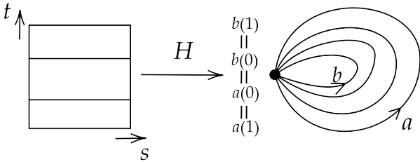
图 10.4: 道路同伦示意图 2
