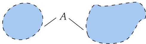
图 7.9: \mathbb{E}^n 的开子集不是道路连通的
