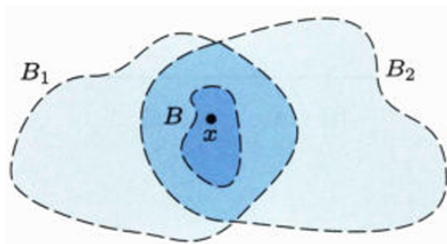
图 2.1: 拓扑基的特性
