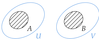
图 5.2: 正规空间
