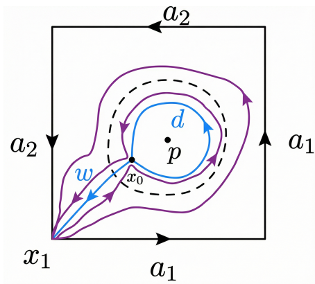
图 10.45: 克莱因瓶的基本群计算
