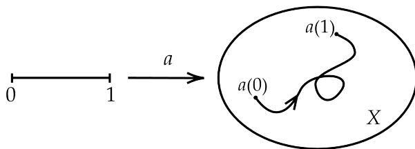
图 7.4: 道路
