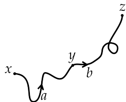
图 7.7: 乘积道路
