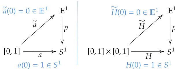
图 10.24: 两个引理的交换图
