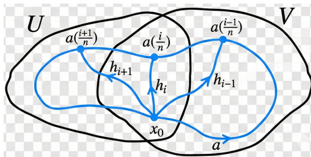
图 10.41: 回路分割示意图
