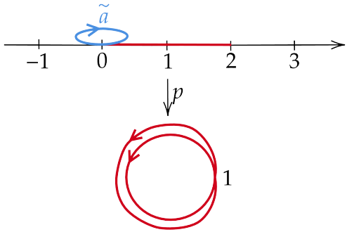
图 10.28: 满射性示意图
