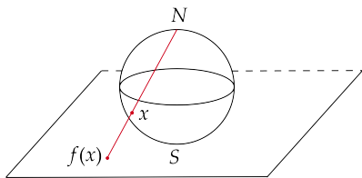
图 3.3: 球极投影示意图
