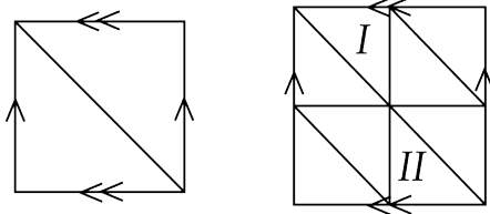
图 9.14: 两个错误的 T^2 的三角剖分
