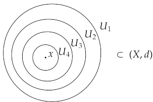
图 5.5: 可数邻域基
