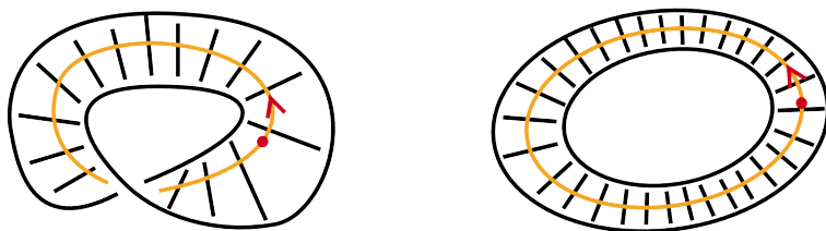
图 9.5: 不可定向曲面与可定向曲面
