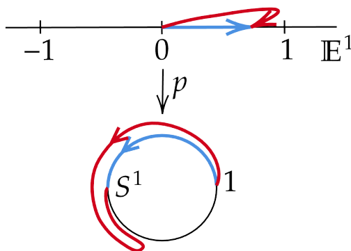
图 10.26: 基本群的同构
