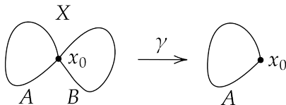
图 10.32: 收缩示例
