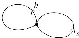
图 10.7: 乘积道路示意图 2
