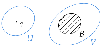
图 5.1: 正则空间
