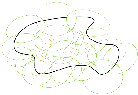
图 6.2: Lebesgue 引理示意
