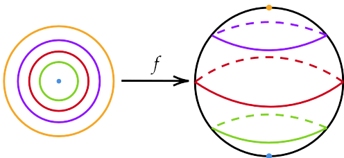
图 8.1: n=2 的情形
