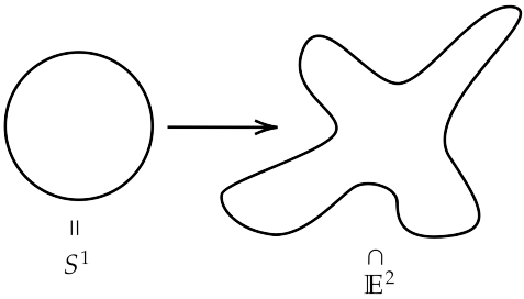
图 3.6: 圆的嵌入
