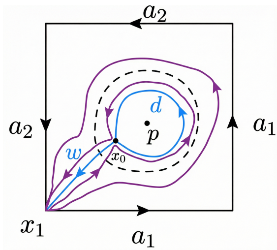
图 10.45: 克莱因瓶的基本群计算
