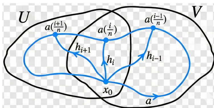
图 10.41: 回路分割示意图
