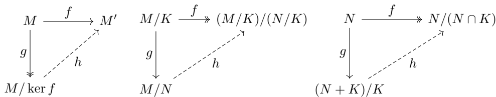
图 3.1: 证明示意.
