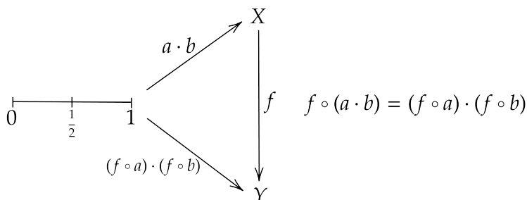
图 10.17: 证明图例
