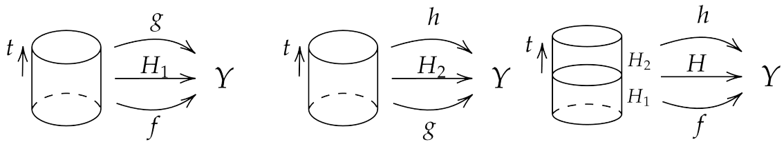
图 10.2: 同伦的传递性
