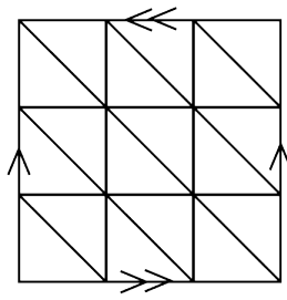
图 9.16: 克莱因瓶的三角剖分
