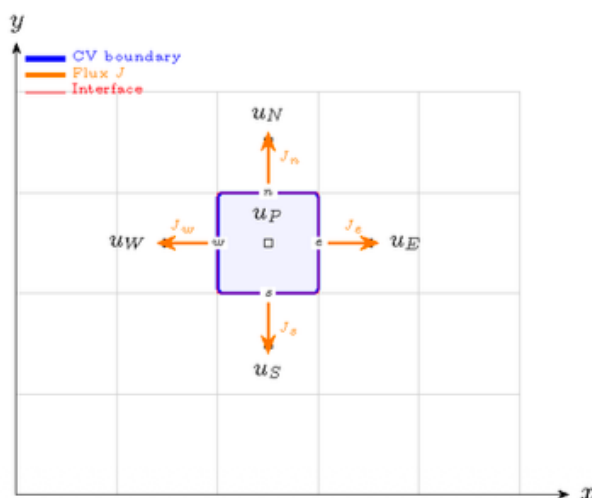
图 2.5: 求解 Poisson 方程的有限体积法网格示意图
