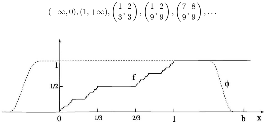
图 8.1: Cantor 函数 f 及一个检验函数 \phi ，表明 g(x) \equiv 0 不可能是 f 的弱导数.
