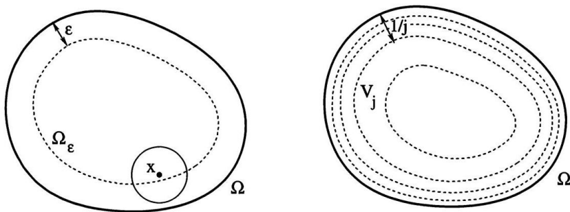
图 8.2: 左: 到边界距离 > \varepsilon 的点构成的开子集 \Omega_\varepsilon \subset \Omega ; 右: 区域 \Omega 可被可数个开子域 V_j = \Omega_{1/(j-1)} \setminus \overline{\Omega}_{1/(j+1)} 覆盖.
