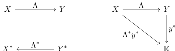
图 4.2: 伴随算子定义中涉及的映射.
