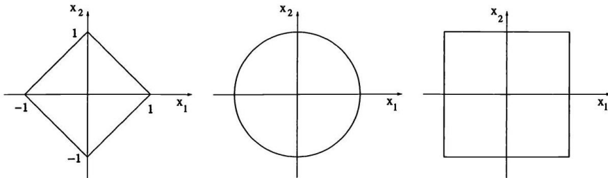
图 2.1: 例 2.2 所述的 \mathbb{R}^2 中单位球，其范数分别为 \|\cdot\|_1 (左)、 \|\cdot\|_2 (中) 和 \|\cdot\|_\infty (右)。
