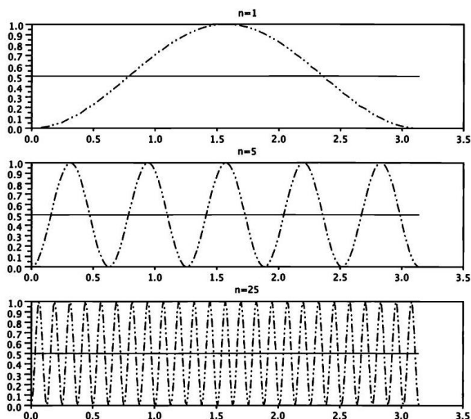
图 5.4: 函数 f_n(x) = \sin^2 nx 的图像 ( n 取 1、5、25). 当 n \rightarrow \infty 时, 函数 f_n 既不逐点收敛, 也不按 L^2 范数收敛. 然而, 我们有弱收敛 f_n \rightharpoonup f \equiv 1/2 , 因为 f_n 在任意区间 (a, b) 上的平均值均收敛于常数 1/2 .
