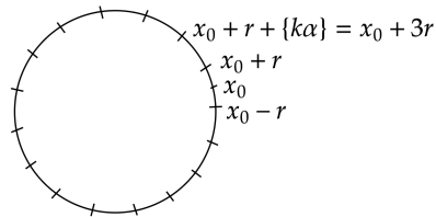
图 2.6: R_{k\alpha} 作用在区间上
