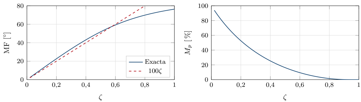
Figura 9: Margen de fase y sobrepeco en función de \zeta para el segundo orden estándar.
