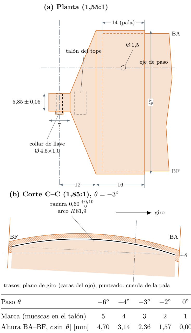
Figura 12.6: Plano F2: portapala. (a) Planta: ojo de bisagra con collar de llave, cuello, encastre de 16 mm con la pala pegada en 14 mm y pasador de ubicación \varnothing 1,5 mm al 25 % de la cuerda, que fija la posición radial de la pala. La ranura se desplaza 0,36 mm hacia el eje respecto del anteproyecto (sección 12.5). (b) Corte por el encastre: ranura curva del radio de la pala, girada \theta alrededor del eje de paso respecto de las caras del ojo; borde de ataque abajo para \theta < 0 . Tolerancia de \theta : \pm 0,2^\circ ; se verifica con la altura BA–BF sobre mármol.
