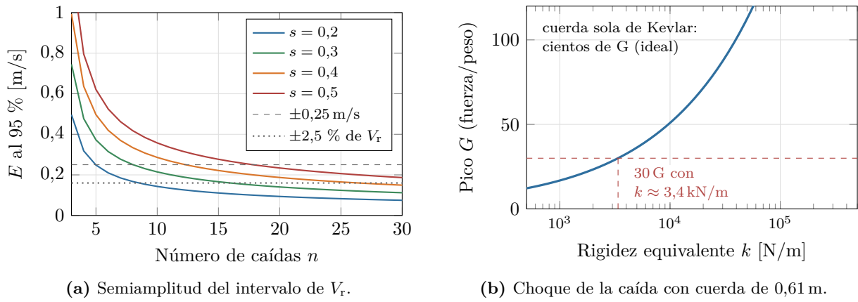
Figura 16.4: (a) Caídas necesarias según la dispersión s [m/s]. (b) Pico de aceleración en función de la rigidez de toda la cadena cuerda–soporte–CanSat (ec. 16.11).
