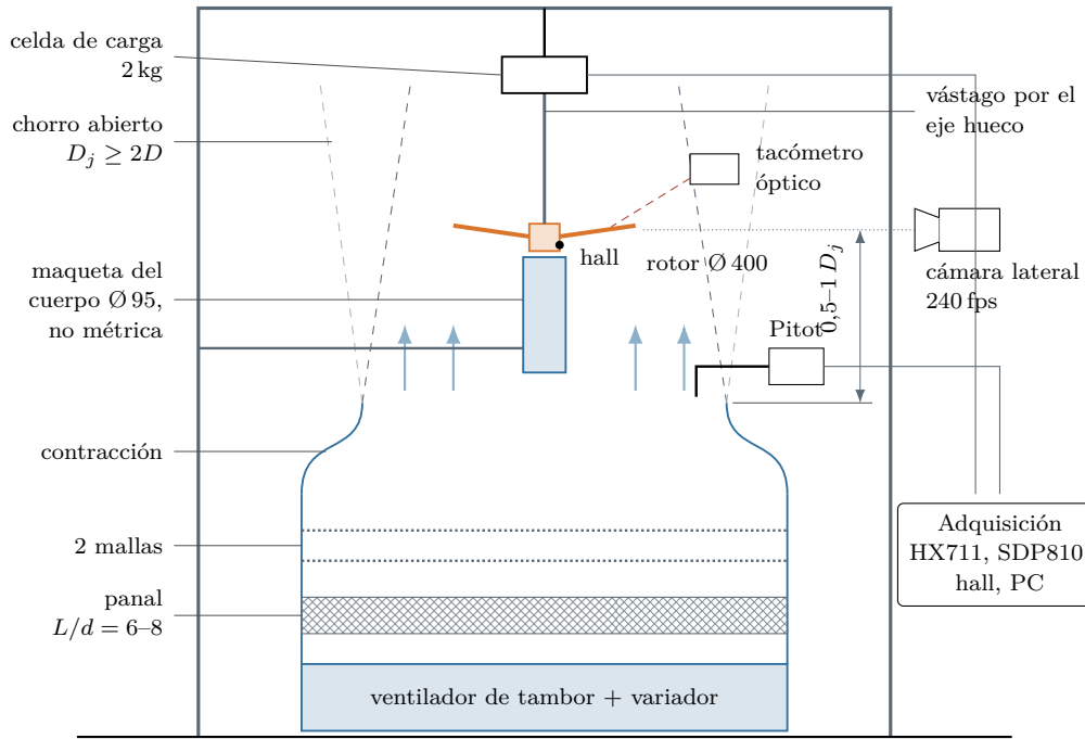
Figura 16.1: Banco vertical de chorro abierto (esquema, sin escala). Naranja: rotor; azul: partes fijas; rojo punteado: haz del tacómetro óptico.
