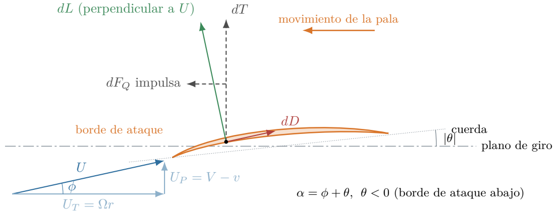
Figura 5.2: Triángulo de velocidades y fuerzas en una sección de pala de un rotor libre en descenso. El aire llega desde abajo y desde adelante; la sustentación queda inclinada hacia adelante y es la que impulsa el giro.
