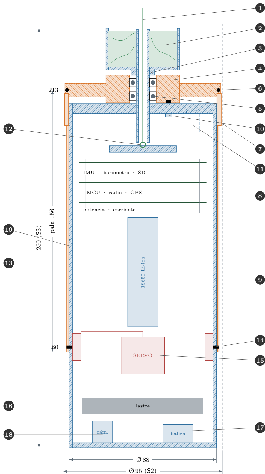
Figura 10.1: Plano 1: conjunto plegado, configuración A, corte longitudinal por el plano de dos palas opuestas (escala aproximada 3:4). Las referencias se listan en la tabla 10.1.
