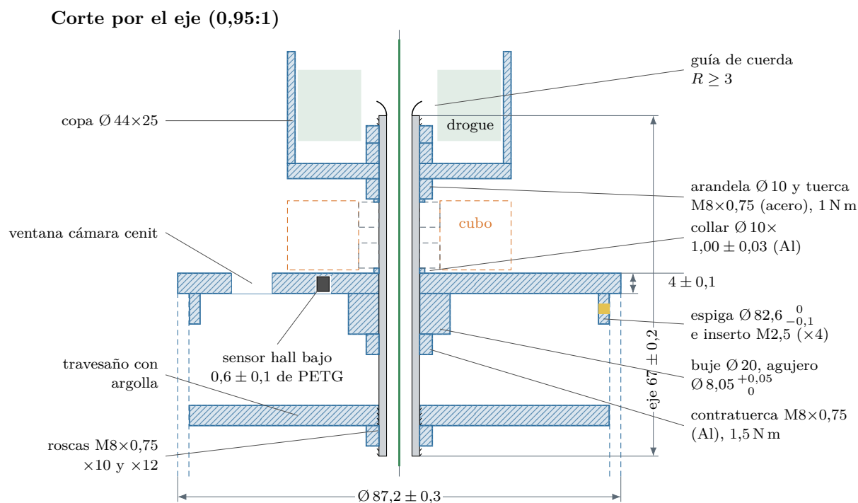
Figura 12.11: Plano F6: tapa superior con eje fijo, travesaño y cabeza del rotor (cubo y rodamientos en trazos). La pila interior (collar, aros interiores, separador, arandela y tuerca de retención, todos de Ø 10 mm como máximo) se aprieta contra la cara de la tapa: el collar es el hombro inferior que pide el capítulo 11. El rodamiento inferior es el fijo y el superior, el libre. El eje hueco lleva roscas M8×0,75 en ambos extremos; la rosca deja 1,0 mm de pared en el fondo del filete, suficiente para las cargas de aterrizaje (106 N) pero no para apretar de más.
