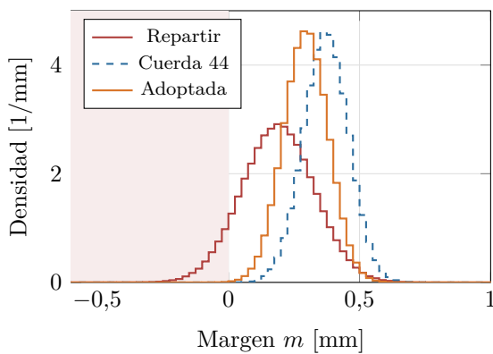
(a) Distribución del margen de envolvente.
