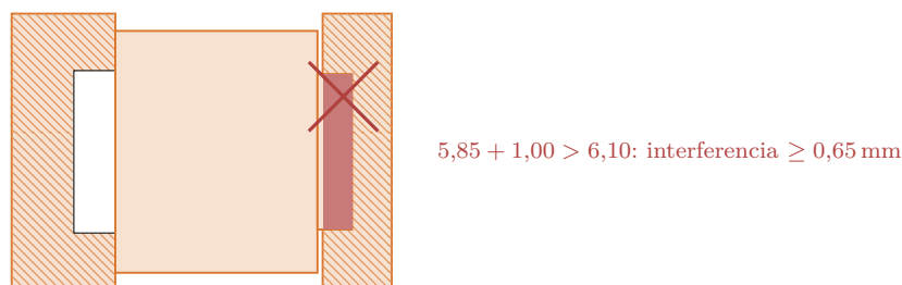
Figura 12.7: Plano F3: horquilla del cubo y llave del portapala. (a) Montaje correcto: el collar entra en la caja de la oreja ancha y el ojo apoya en las caras de la ranura; el collar nunca toca el fondo de la caja. (b) Dado vuelta, el collar choca con la oreja angosta y el pasador no puede pasar. El pasador se coloca a presión desde la oreja ancha.
