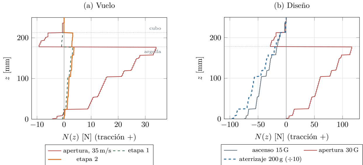
Figura 11.6: Esfuerzo axial a lo largo del eje del CanSat, ecuación (11.4) (datos en planos_axial.dat ). El salto en z = 178 mm es la cuerda; el de z = 213 mm, el empuje del rotor. Arriba de la argolla la pieza trabaja en compresión al abrir el drogue: el cubo y la copa apoyan hacia abajo.
