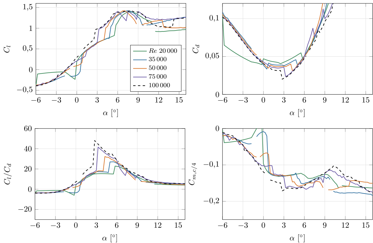
Figura 7.3: Placa curvada al 7% ( t = 1,5\% ), XFOIL con N_{\text{crit}} = 9 : C_l , C_d , C_l/C_d y C_m respecto de c/4 en función de \alpha . Los huecos son ángulos sin solución convergida.
