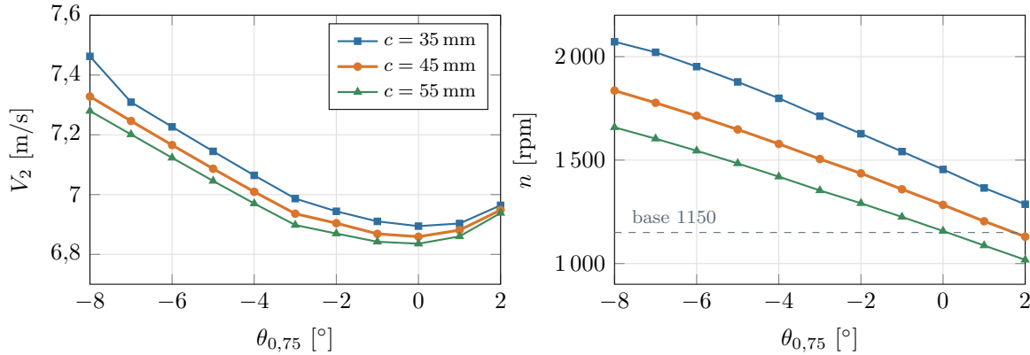
Figura 8.4: Efecto del paso y de la cuerda ( B = 4 , con drogue).
