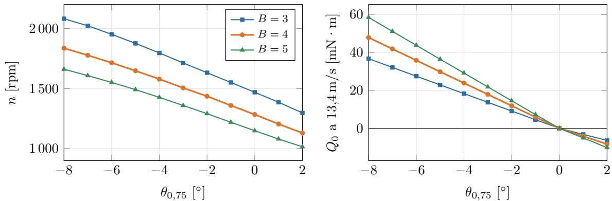
Figura 8.5: Efecto del número de palas ( c = 45 mm): rpm de equilibrio y par de arranque a \Omega = 0 .
