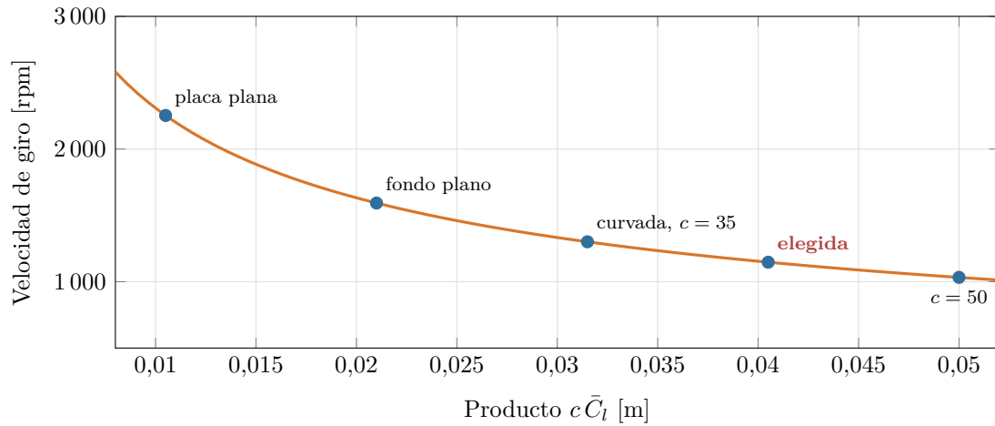
Figura 6.3: La velocidad de giro baja con la raíz de c\bar{C}_l (con el mismo empuje y la misma velocidad de caída).
