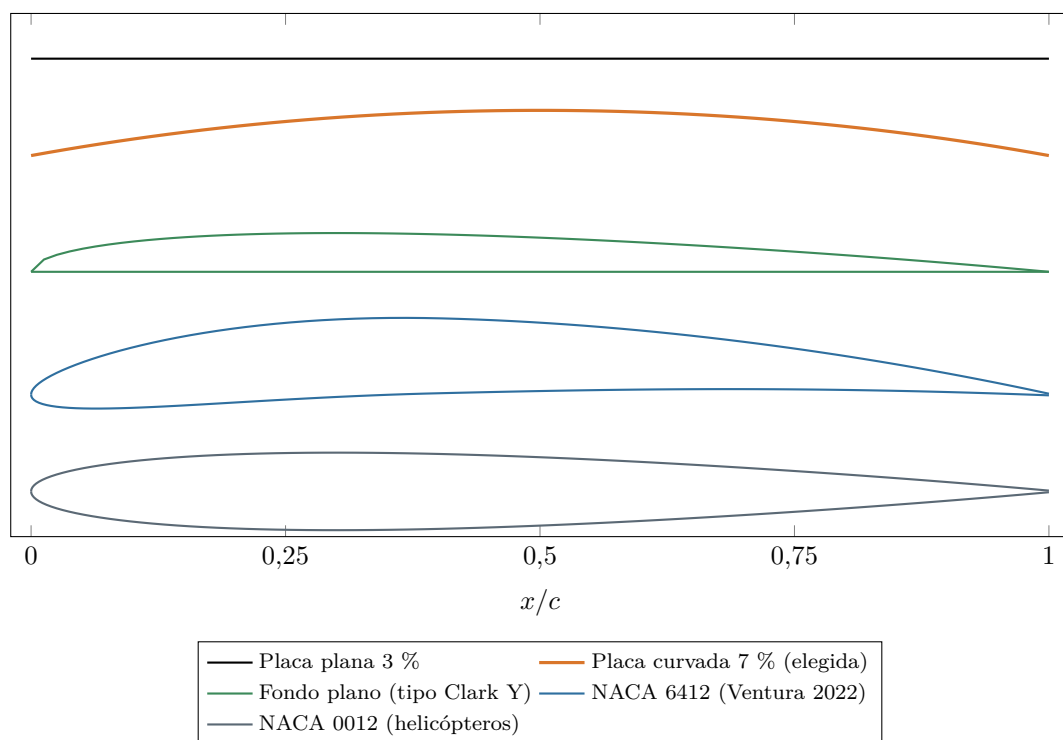
Figura 5.4: Secciones comparadas, desplazadas en vertical para verlas por separado. La escala vertical está ampliada unas 2,5 veces respecto de la horizontal. El espesor de la placa curvada se dibuja como una línea porque es el 1,1 % de la cuerda.
