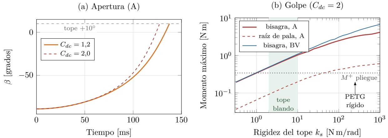
Figura 9.4: (a) Ángulo de batimiento durante la apertura de la pala A: recorre 99^\circ en 127 ms–138 ms. (b) Momento máximo en la bisagra (reacción del tope) y en la raíz de la pala tras el golpe, en función de la rigidez del tope. Un tope de PETG con contacto de 4 \times 2 mm a 4 mm del pasador tiene k_s \approx 250 N m/rad.
