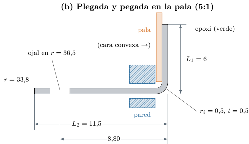
Figura 12.10: Plano F5, hoja (b): pestaña plegada y pegada sobre la cara convexa de la punta de la pala; el ala radial pasa por la ranura de la pared (huelgos exagerados).
