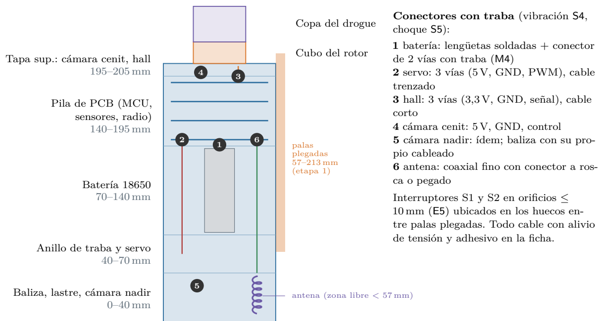
Figura 14.2: Arnés y conectores sobre la distribución de alturas de la tabla 6.9 (escala vertical comprimida). En la etapa 1 las palas de carbono, conductoras, cubren el cuerpo entre 57 y 213 mm; la antena debe quedar debajo.
