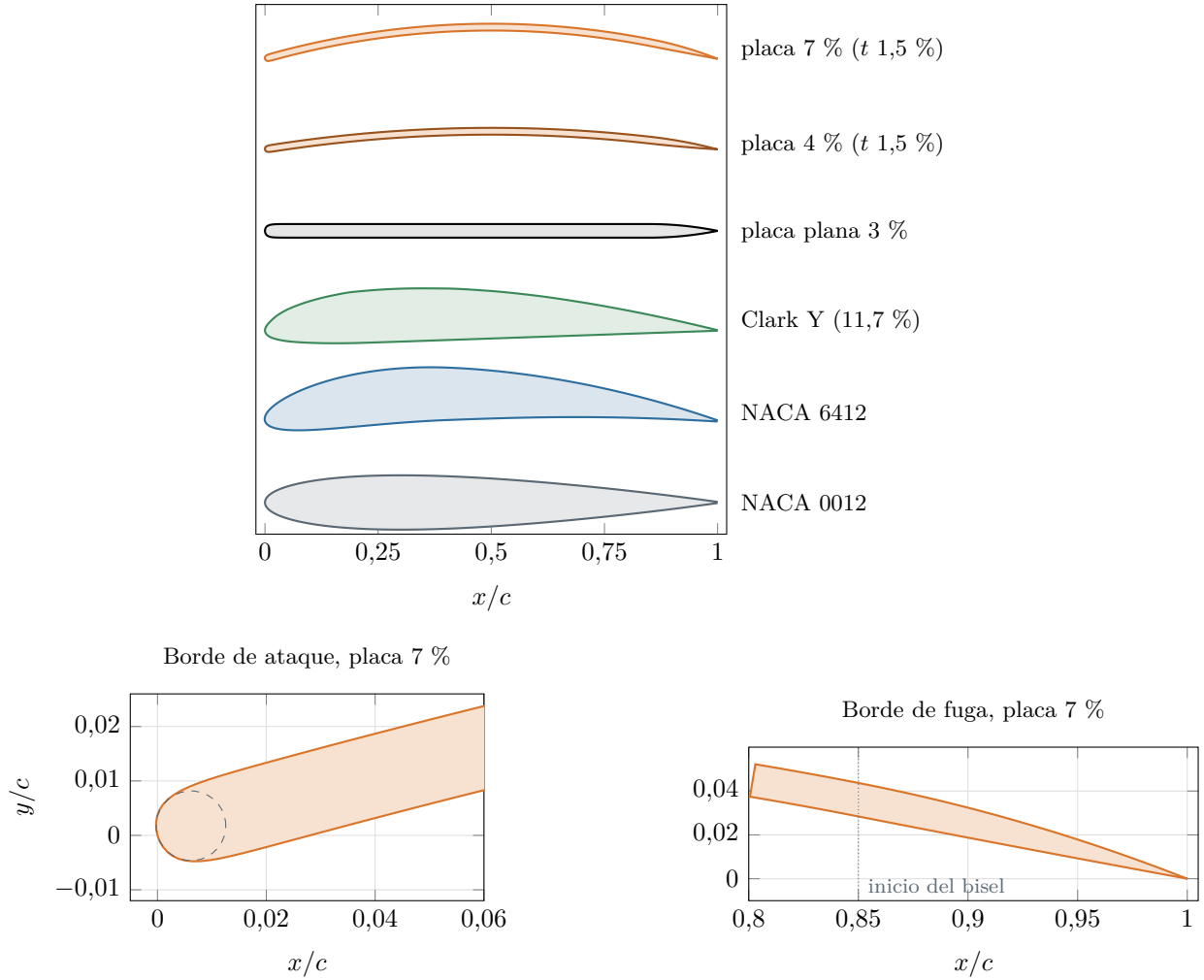
Figura 7.2: Arriba: las seis secciones a escala real (cuerda unitaria), desplazadas en vertical. Abajo: detalle de la nariz semicircular (círculo de trazos de radio 0,0064c ) y del bisel de fuga del modelo de la placa al 7%.
