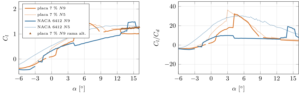
Figura 7.7: Sensibilidad a N_{\text{crit}} a Re = 50\,000 . Los triángulos son la segunda solución de los ángulos biestables de la placa al 7 % con N_{\text{crit}} = 9 (rama de C_l alto, no incluida en la polar principal).
