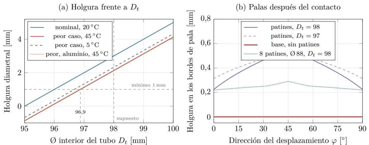
Figura 11.10: (a) Holgura diametral con la ecuación (11.5) (tubo de fibra de vidrio salvo indicación; datos en planos_holgura.dat ). (b) Holgura que queda en los bordes de las palas cuando el cuerpo, desplazado en la dirección \varphi (medida desde el centro de una pala), toca el tubo (datos en planos_seccion.dat ). Las curvas «patines» son la propuesta con cuerpo Ø 87. Sin patines la holgura es cero en todas las direcciones: el contacto es la pala.
