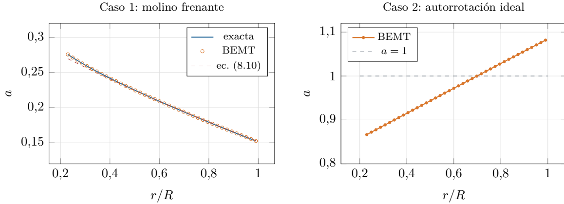
Figura 8.2: Validación del código BEMT con dos casos de referencia.
