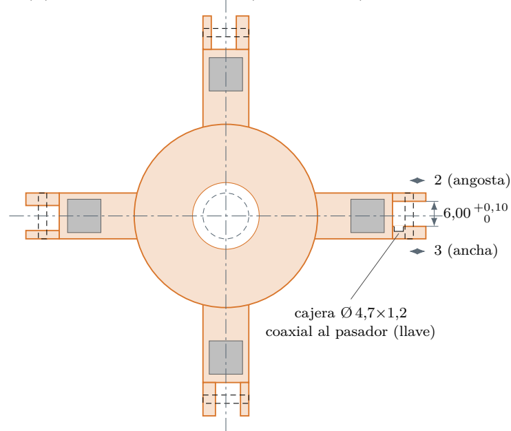
(b) Planta desde arriba (escala 0,8:1)
