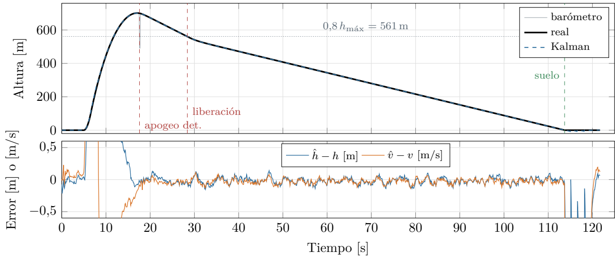
Figura 14.3: Vuelo nominal en lazo cerrado (escenario 2). La lógica C detecta el apogeo 0,52 s después del real y libera a 560,5 m (79,9 % de 701,4 m), a 0,04 s del cruce real del 80 %. En el ascenso rápido el error llega a 15 m y 9 m/s (fuera de escala) por el error de presión dinámica supuesto (hasta 8 m): la compuerta rechaza esas lecturas hasta el re-anclaje (sin compuerta el error de altura sería de 9 m). El error desaparece antes del apogeo: cerca de él es de 0,11 m y 0,29 m/s, y en todo el descenso queda por debajo de 0,15 m y 0,14 m/s. El pico final (7 m, 6,5 m/s) aparece al tocar el suelo: el choque del impacto se descarta como el de la expulsión, el filtro sigue «bajando» y la compuerta rechaza el barómetro hasta re-anclar.
