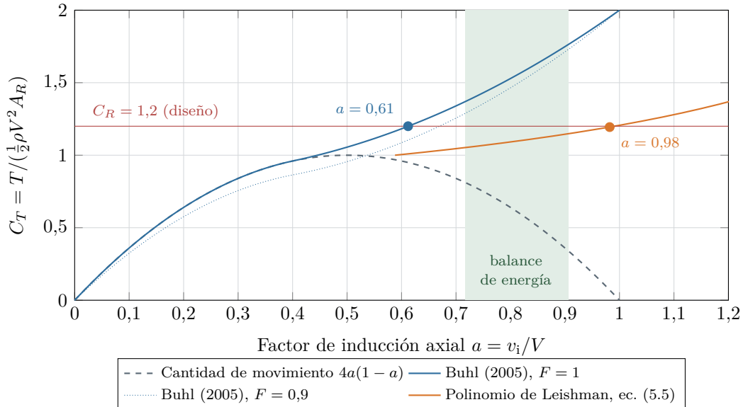
Figura 4.3: Coeficiente de empuje frente a factor de inducción: dos curvas empíricas de origen distinto (turbinas y helicópteros) dan factores de inducción muy diferentes para el C_R de diseño. La franja verde es el rango de a que pide el balance de energía de la tabla 4.5 (estimación). Datos: analysis/data/literatura_ct_*.dat .
