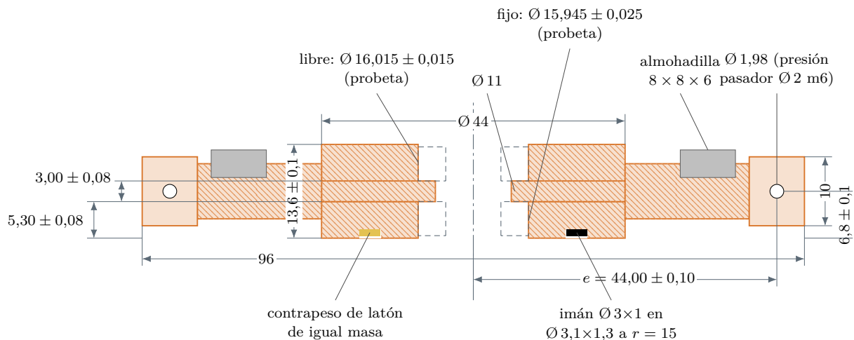
Figura 12.4: Plano F1, hoja (a): cubo en corte. Asiento inferior (rodamiento fijo) con interferencia calibrada y asiento superior (libre) deslizante; nervio central de 3,00 mm que apoya sobre el rodamiento fijo y le transmite las cargas hacia abajo; orejas de la bisagra a e = 44 mm, almohadilla de silicona del tope de 15^{\circ} e imán del sensor hall con su contrapeso.
