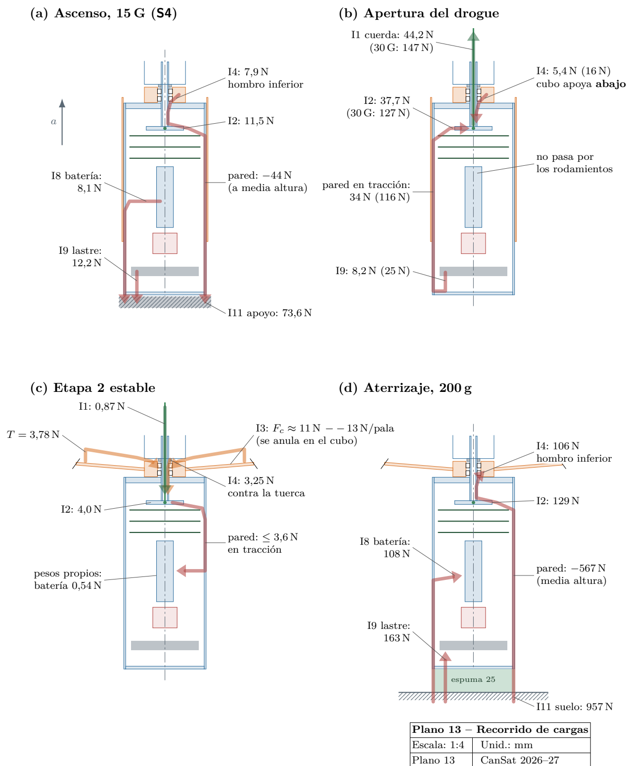
Figura 11.5: Plano 13: recorrido de cargas en cuatro casos (corte simplificado a escala 1:4). Las franjas indican el camino de la carga y su sentido de transmisión; los números son fuerzas en cada interfaz (tabla 11.4). En (b), entre paréntesis, el caso de diseño de 30 G (S5). Palas desplegadas recortadas en (c) y (d). En (d) el anillo de espuma de 25 mm del capítulo 9 se dibuja bajo la tapa inferior; para respetar los 250 mm de S3 ese capítulo lo ubica a costa del tramo de baliza y lastre, cambio que los planos 9, 11 y 15 todavía no reflejan. Valores estimados con (11.4).
