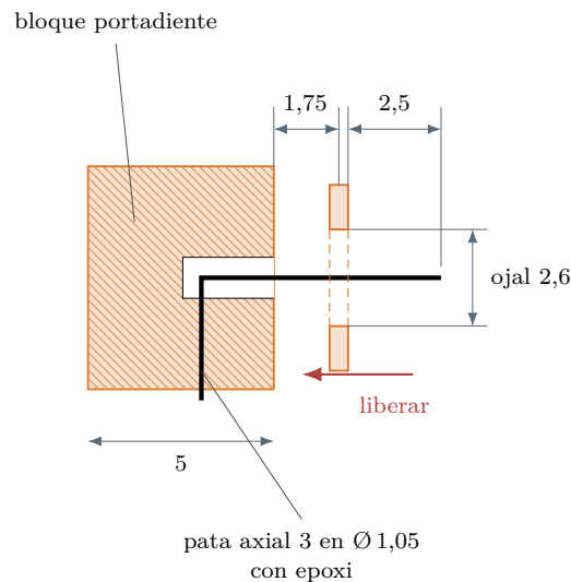
Figura 12.8: Plano F4: anillo de traba. (a) Planta en posición trabada: anillo PETG R 26-32 de 4 mm de alto, cuatro bloques portadiente y dientes de alambre Ø 1,0 mm a R = 36,5 mm que atraviesan las pestañas. El talón del anillo apoya en un tope fijo en la posición trabada. (b) Detalle desarrollado sobre R = 36,5 (horizontal: arco; vertical: dirección del eje): enganche de 2,5 mm más allá de la pestaña y ojal colisado de 2,6 mm en la dirección del eje.
