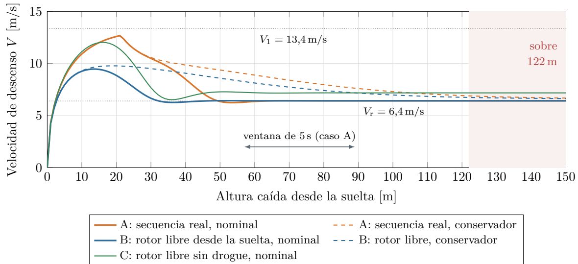
Figura 16.3: Velocidad en función de la altura caída, según el modelo de orden reducido (16.6)–(16.7). En el caso A el rotor se libera a los 2,5 s ( V \approx 12,7 \text{ m/s} ). Zona roja: por encima del límite de la categoría abierta [133].
