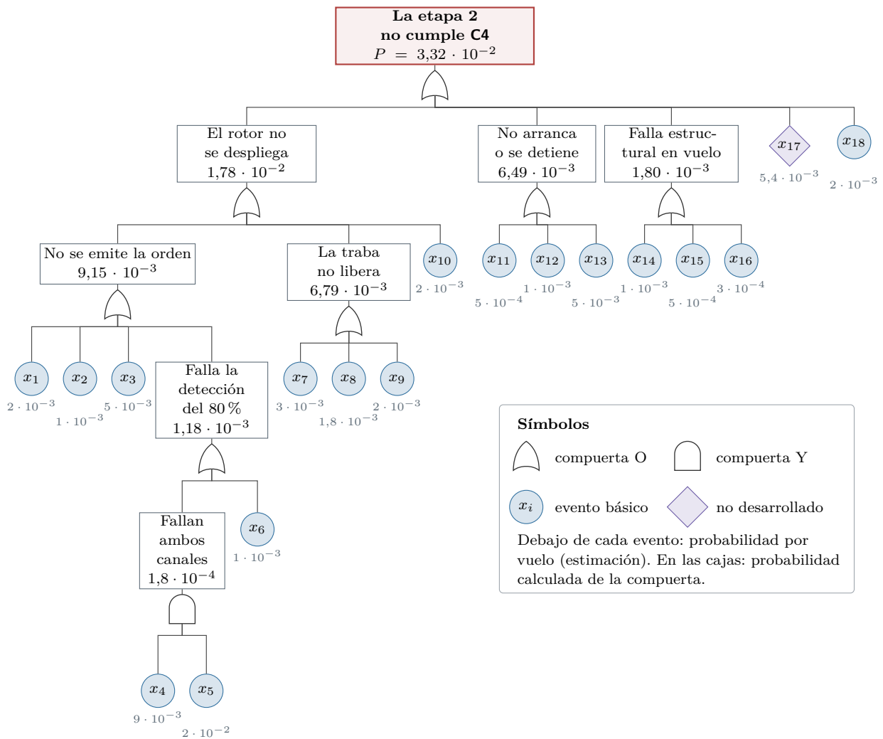
Figura 17.1: Árbol de fallas del evento “la etapa 2 no cumple C4”. Los códigos x_i se describen en la tabla 17.2. x_{17} no se desarrolla en el árbol: se calcula por Monte Carlo (sección 17.2.1).
