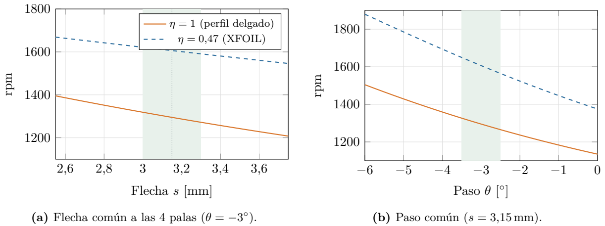
Figura 12.1: Sensibilidad de la velocidad de giro a la flecha y al paso (modelo (12.3)–(12.4), solo relativo). Banda verde: tolerancia adoptada ( \pm 0,15 mm; \pm 0,5^\circ ).
