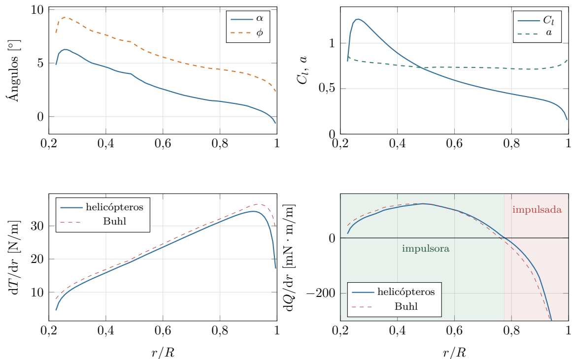
Figura 8.3: Distribuciones radiales en el punto de diseño ( \theta = -3^\circ , 80 anillos). El área de dQ/dr es nula: equilibrio de par.
