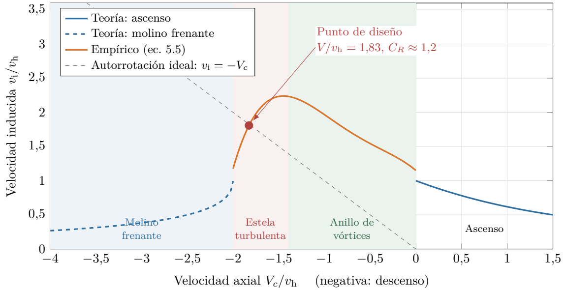
Figura 5.1: Velocidad inducida en vuelo axial. La teoría de cantidad de movimiento vale en ascenso y en el estado de molino frenante; entre ambos se usa la curva empírica. El rotor libre opera cerca de la autorrotación ideal, donde el flujo neto a través del disco es casi nulo ( V_c + v_i \approx 0 ).
