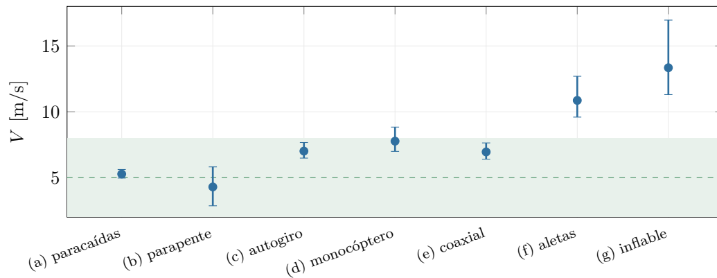
Figura 18.2: Velocidad de la etapa 2 con el sistema funcionando: mediana e intervalo del 90 % (Monte Carlo). La banda verde es C4.
