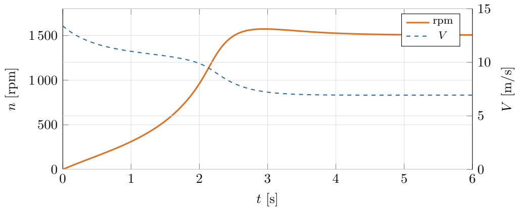
Figura 8.10: Arranque cuasiestacionario desde \Omega = 0 y V = 13,4 \text{ m/s} ( \theta = -3^\circ , con drogue).
