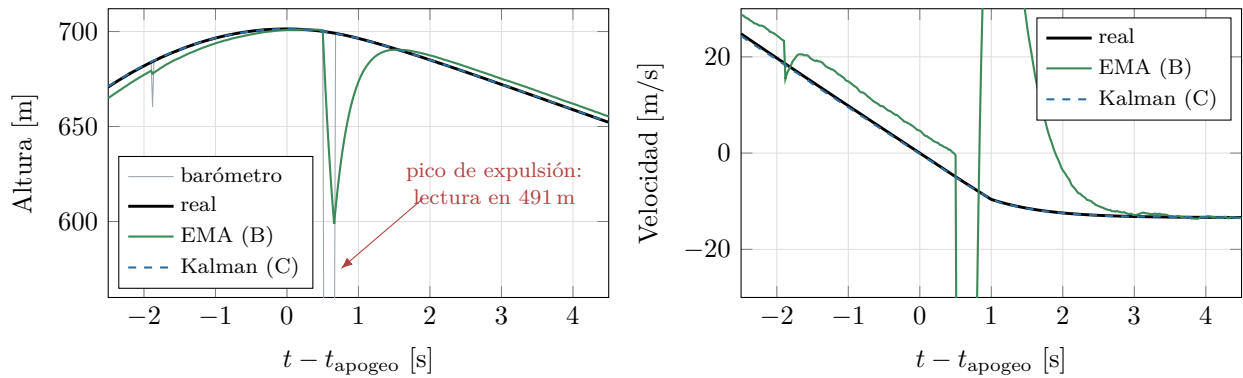
Figura 14.4: Detalle del apogeo y de la expulsión (a +0,52 s) del vuelo nominal. El pico de 2,5 kPa lleva la lectura cruda a 491 m, por debajo del umbral de 561 m: la lógica A libera en ese instante a 700 m. La EMA baja hasta 599 m y su velocidad hasta -299 m/s (fuera de escala). El filtro C rechaza las muestras del pico y no se aparta de la altura real.
