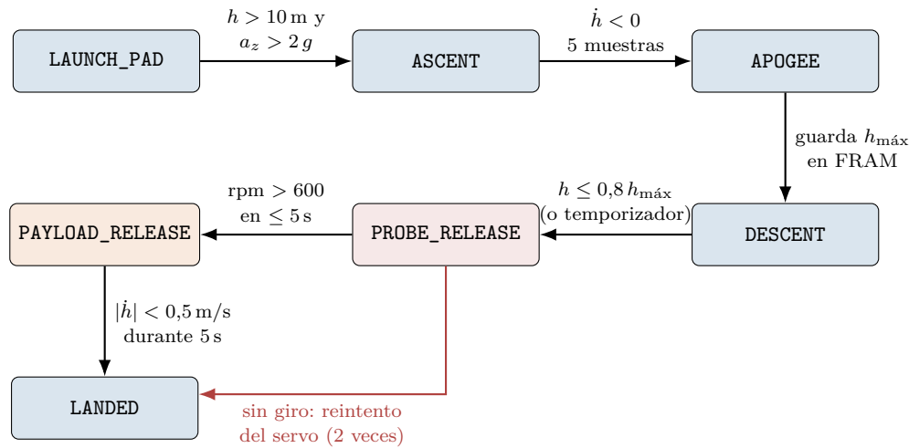
Figura 13.2: Máquina de estados del software de vuelo con las transiciones propuestas. Los umbrales son valores iniciales a ajustar en ensayo.
