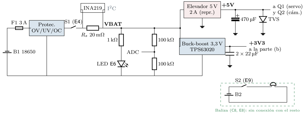
(a) Potencia: celda, protección, interruptor, medición y rieles.
