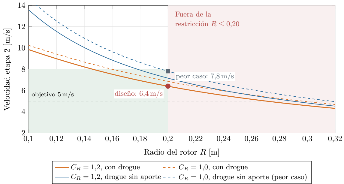
Figura 6.2: Velocidad de la segunda etapa en función del radio. Con R = 0,20 m todos los casos quedan bajo 8 m/s; llegar a 5 m/s exactos pediría R \approx 0,27 m.
