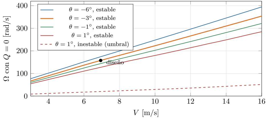
Figura 8.9: Lugar de equilibrio de par Q(\Omega, V) = 0 . Con \theta = 1^\circ aparece una raíz inestable a bajas rpm que hace de umbral: por debajo de ella el rotor se frena.
