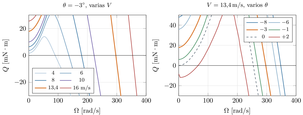
Figura 8.8: Curvas de par Q(\Omega) . Izquierda: paso recomendado a distintas velocidades. Derecha: distintos pasos a la velocidad de la etapa 1.
