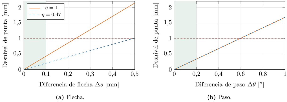
Figura 12.2: Desnivel de la punta de una pala respecto de las otras tres, por ecuación (12.5). Línea roja: límite de 1 mm (0,5 % de R ) adoptado para el banco. Banda verde: dispersión admitida en el juego. En (b) las dos curvas coinciden: el desnivel por paso no depende de \eta .
