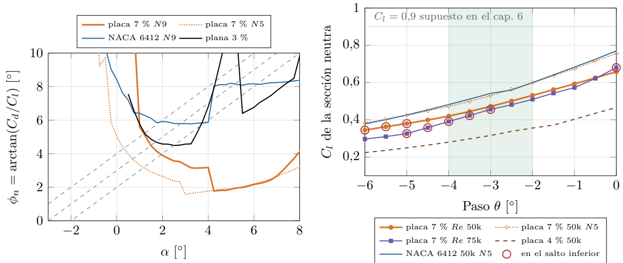
Figura 7.11: Sección neutra en autorrotación (ec. 7.11). Izquierda: la solución es el cruce de \phi_n(\alpha) con la recta \alpha - \theta (trazos grises; de arriba hacia abajo \theta = -4^\circ , -3^\circ y -2^\circ ). Derecha: C_l de la solución en función del paso; la banda verde es el paso recomendado.
