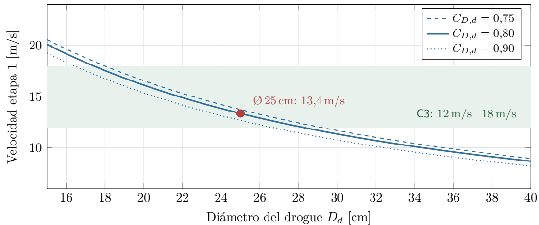
Figura 6.1: Velocidad de la primera etapa según el diámetro del drogue (incluye el cuerpo).
