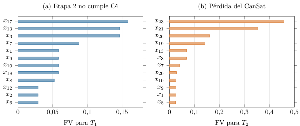
Figura 17.3: Importancia de Fussell–Vesely de los doce eventos básicos más importantes de cada árbol.
