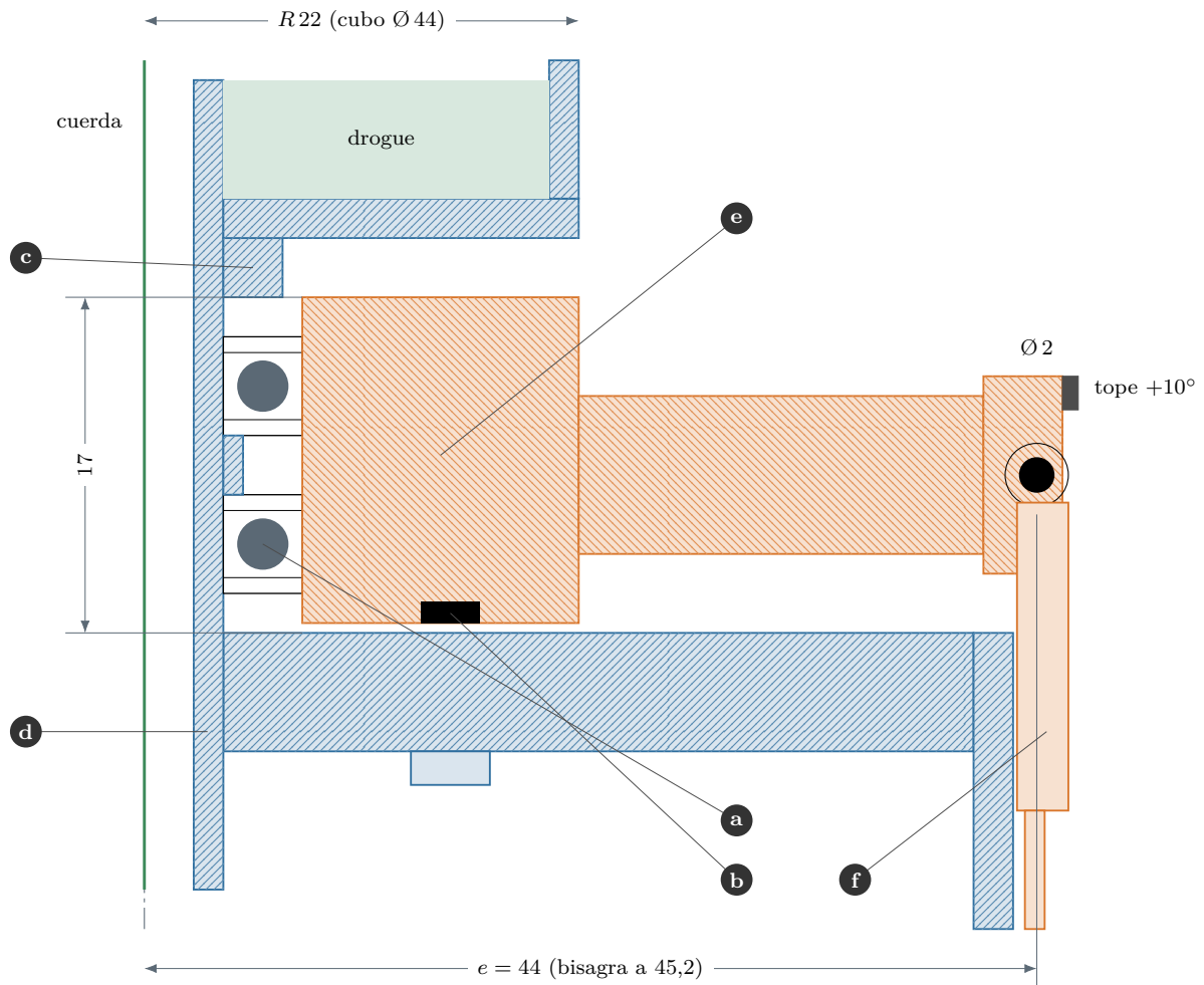
Figura 10.5: Plano 4: detalle del cubo, medio corte (escala aproximada 2,5:1). (a) rodamientos 688ZZ con separador; (b) imán de neodimio y sensor hall; (c) tuerca M8 fina; (d) eje fijo hueco \varnothing 8 \times 5 ; (e) cubo giratorio; (f) portapala con la pala colgando. La sustentación empuja el cubo hacia arriba contra la tuerca; el tirón del drogue va por la cuerda al travesañ de anclaje y no pasa por los rodamientos.
