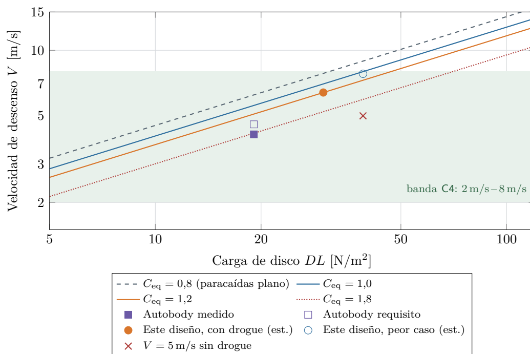
Figura 4.2: Velocidad de descenso frente a carga de disco. Las rectas son C_{eq} constante. Solo se grafican casos con datos publicados completos.
