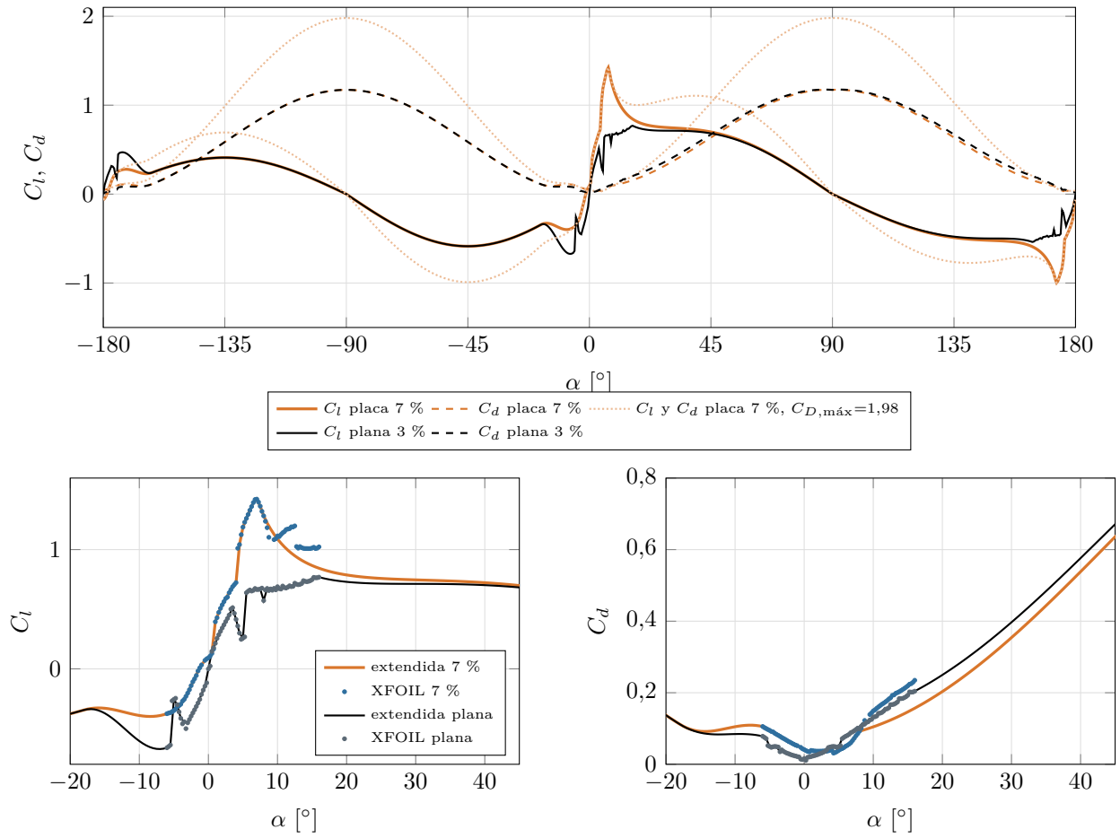
Figura 7.10: Polares extendidas a Re = 50\,000 . Arriba: intervalo completo, con la variante bidimensional ( C_{D,m\acute{a}x} = 1,98 ) de la placa al 7 %. Abajo: detalle del empalme; los puntos son XFOIL (todos los convergidos, incluidos los de post-pérdida que el modelo descarta).
