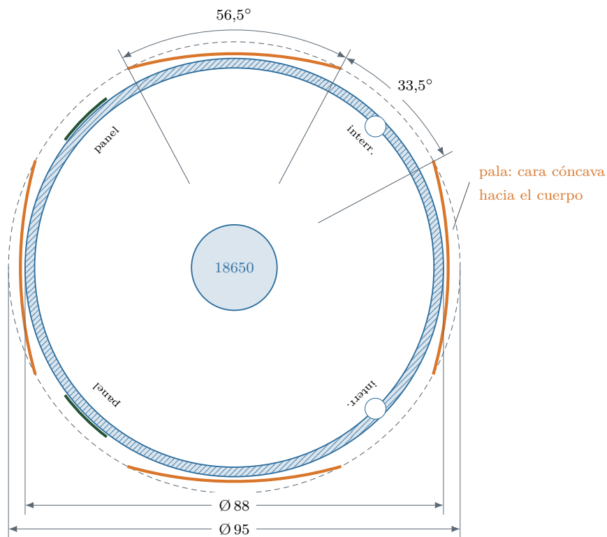
Figura 10.4: Plano 3: corte A–A a media altura con las palas plegadas (escala aproximada 1:1). Cada pala ocupa 56,5°; en los cuatro huecos de 33,5° van los interruptores (E4, E5) y los paneles solares (E3). Los bordes de las palas tocan la envoltura de Ø 95 sin excederla.
