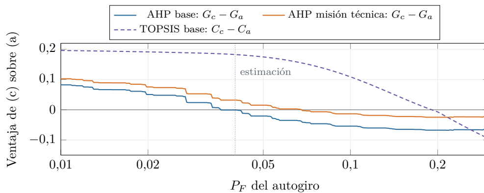
Figura 18.7: Ventaja del autogiro sobre el paracaídas en función de su probabilidad de falla funcional. El autogiro gana mientras la curva esté sobre cero. Las curvas del AHP son escalonadas porque los juicios se redondean a la escala de Saaty.
