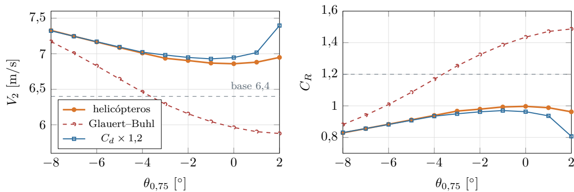
Figura 8.6: Sensibilidad de V_2 y C_R al cierre de cantidad de movimiento y a la resistencia de perfil.
