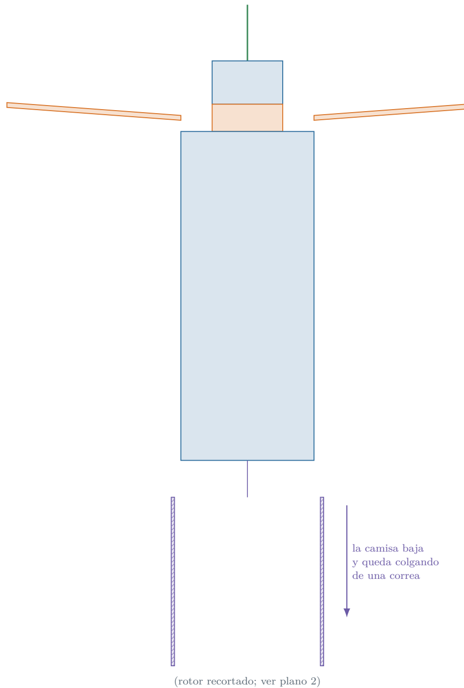
Figura 10.9: Plano 8: configuración B, solo si la organización exige un contenedor que cubra todo el CanSat. La camisa (violeta, pared 2 mm) contiene las palas; al liberarse baja y queda colgando de una correa. Excede el presupuesto de masa en unos 50 g (tabla 6.8).
