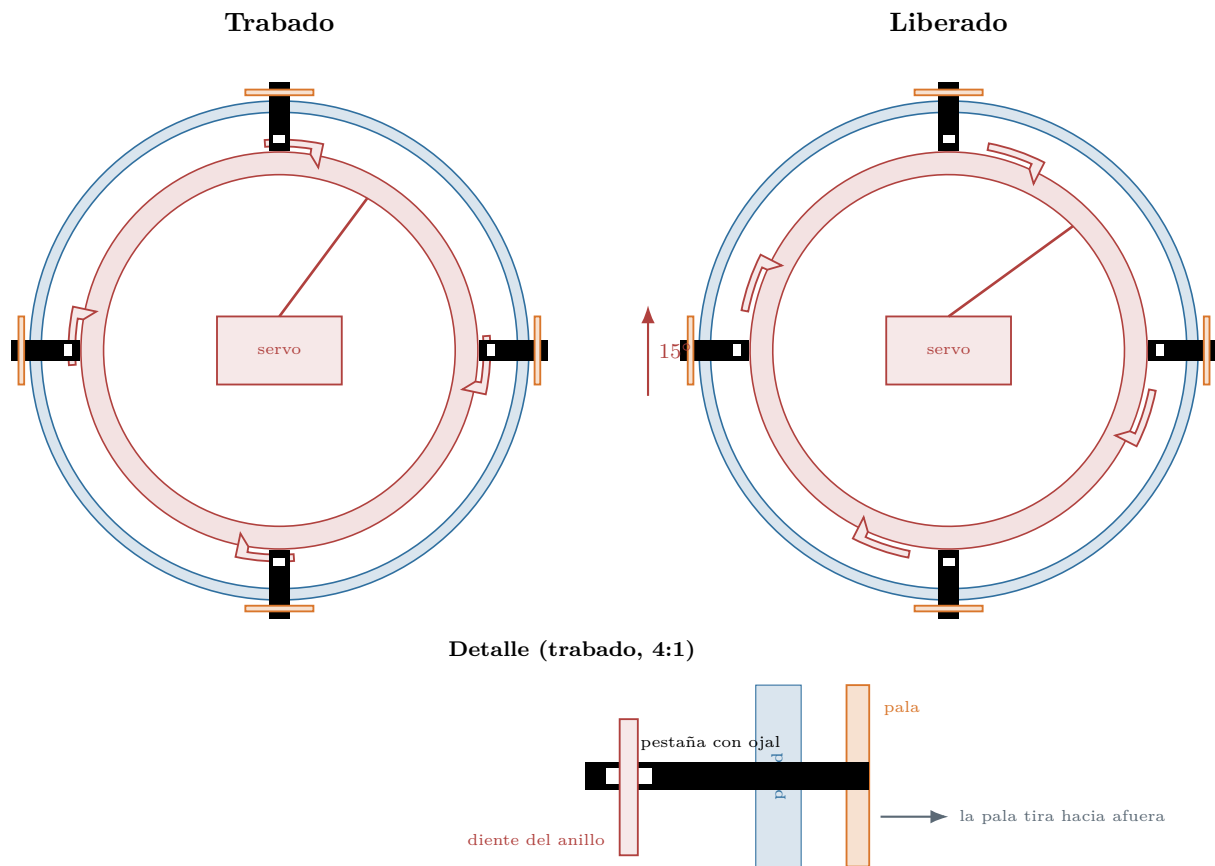
Figura 10.8: Plano 7: anillo de traba, corte B–B a la altura de las pestañas (60 mm del fondo, escala aproximada 3:4). Cada pala termina en una pestaña de acero inoxidable con un ojal, que entra al cuerpo por una ranura de 3 \times 1 mm. Trabado: un diente tangencial del anillo interno pasa por el ojal y la pestaña no puede salir. Liberado: el servo gira el anillo 15^\circ , los cuatro dientes salen de los ojales a la vez y las palas quedan libres. Mecánico, sin calor (M1, M2); el choque no puede girar el anillo (M3).
