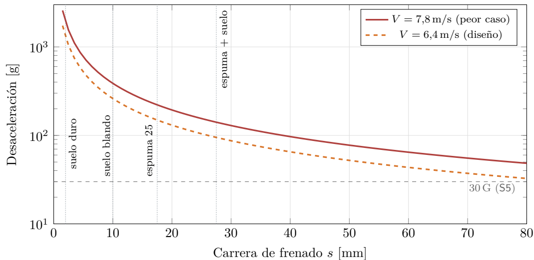
Figura 9.5: Desaceleración de aterrizaje según la carrera de frenado (9.10), con \eta = 0,8 . Las líneas verticales son las carreras supuestas. Bajar a 30 G exigiría 90 mm – 130 mm de carrera, incompatible con S3.
