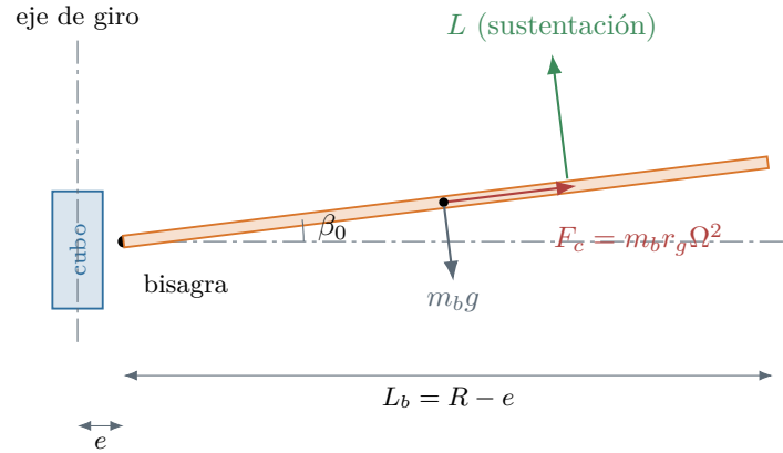
Figura 5.5: Equilibrio de una pala articulada: la sustentación la levanta y la fuerza centrífuga la lleva hacia el plano de giro. El resultado es un ángulo de conicidad \beta_0 de pocos grados.
