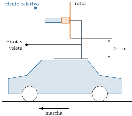
(a) E2b: mástil sobre el auto.
