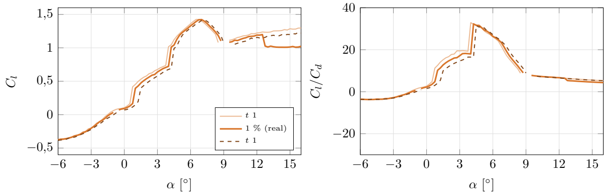
Figura 7.9: Efecto del espesor del modelo de la placa al 7 % a Re = 50\,000 , N_{crit} = 9 .
