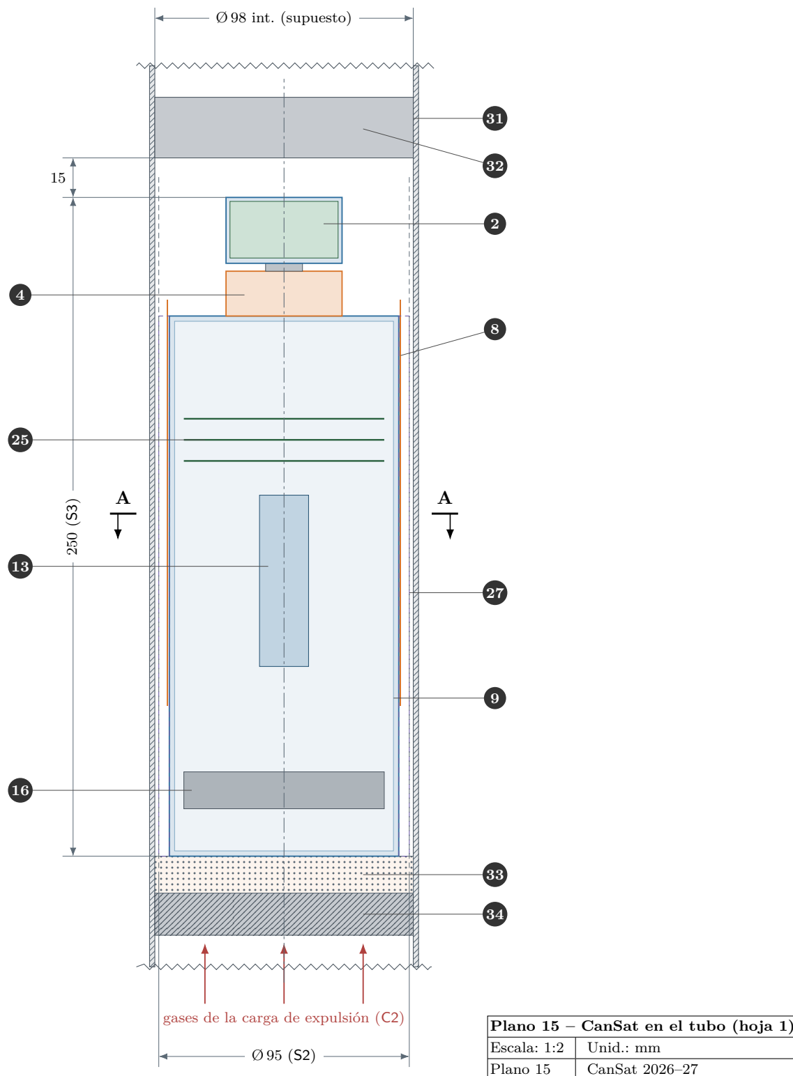
Figura 11.8: Plano 15, hoja 1: corte longitudinal del CanSat plegado dentro del tubo del cohete (escala 1:2). Las palas (8) están cortadas por su plano medio; los patines (27) están a 45° de las palas, fuera del plano de corte (línea de trazos violeta). El tubo (31), la ojiva (32), el protector de gases (33) y la mampara (34) son supuestos : el anexo no los define. Referencias en la tabla 11.6.
