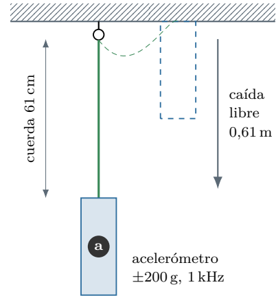
(b) E5b: choque por caída con cuerda [132].
