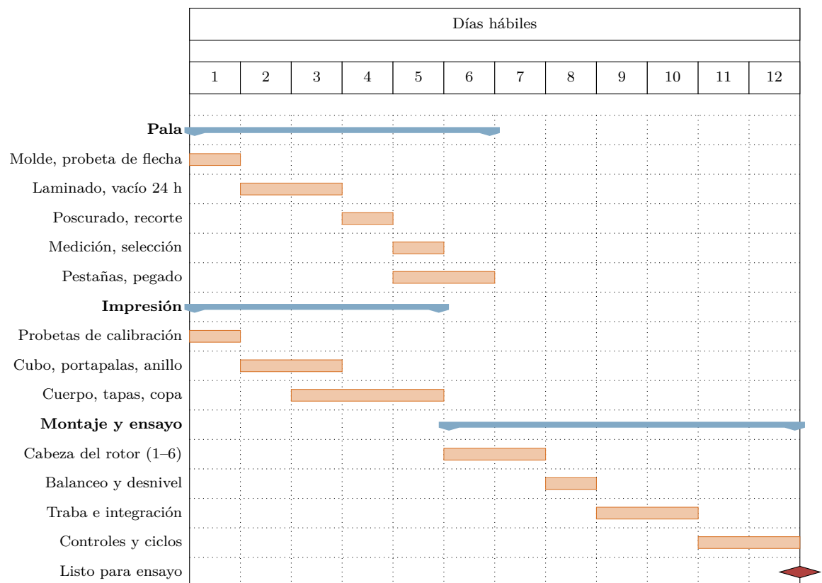
Figura 12.15: Cronograma de fabricación de una unidad de vuelo (estimado).
