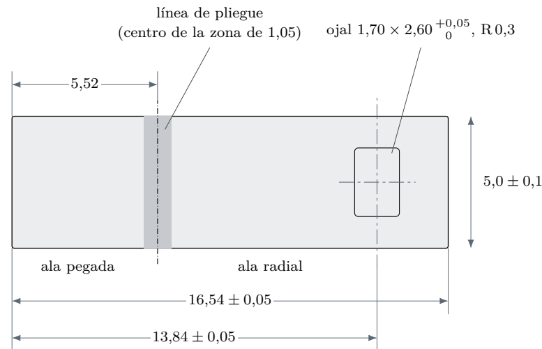
Figura 12.9: Plano F5, hoja (a): desarrollo plano de la pestaña de acero inoxidable AISI 304 de 0,5 mm, según la ecuación (12.10); el ojal se corta en plano, antes de plegar, con una plantilla de acero que referencia el extremo pegado.
