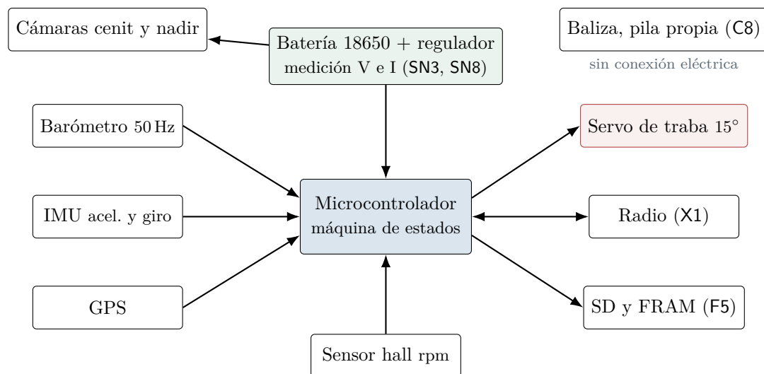
Figura 13.1: Bloques electrónicos relacionados con el descenso. La baliza no comparte alimentación con el resto (C8).
