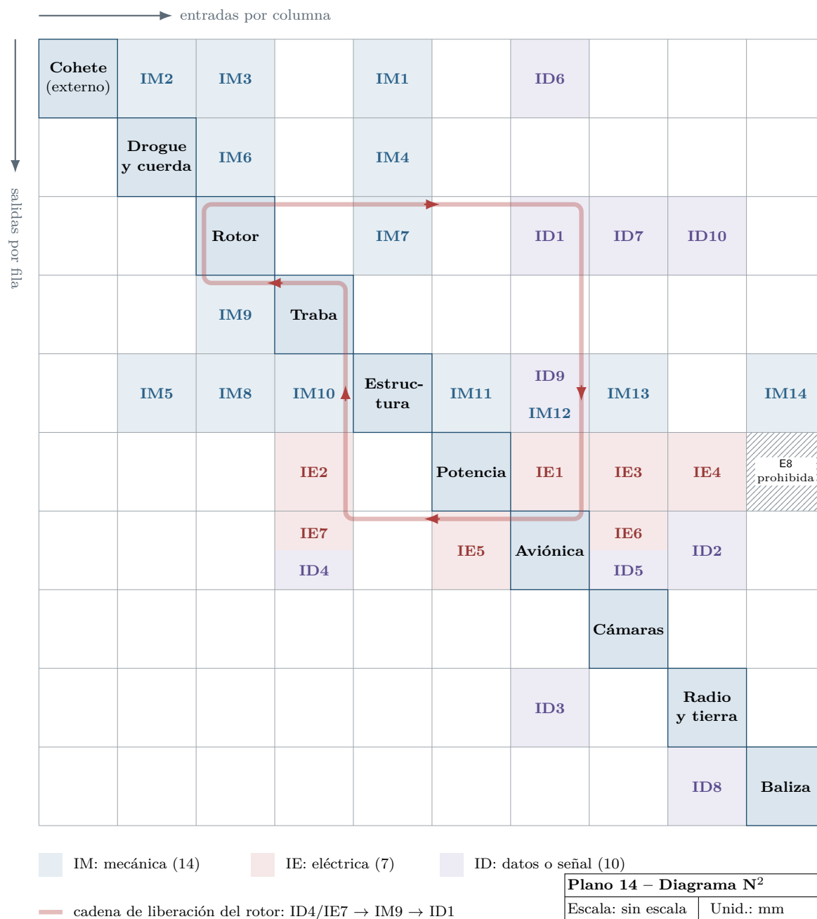
Figura 11.7: Plano 14: diagrama N² de interfaces. Fila i , columna j : lo que el subsistema i entrega al j . La casilla rayada (potencia → baliza) es una interfaz que el anexo prohíbe (E8). La banda roja sigue la cadena que libera el rotor: la aviónica ordena al servo (ID4, IE7), la traba suelta las palas (IM9) y el sensor hall del rotor confirma el giro a la aviónica (ID1). Códigos en la tabla 11.5.
