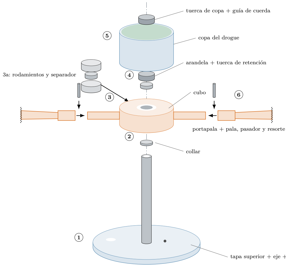
Figura 12.12: Vista explosionada de la cabeza del rotor (perspectiva caballera, escala aproximada 0,6:1; se dibujan dos de las cuatro palas, cortadas). Azul: piezas fijas; naranja: piezas que giran; gris: rodamientos y piezas metálicas. Los números son los pasos de montaje.
