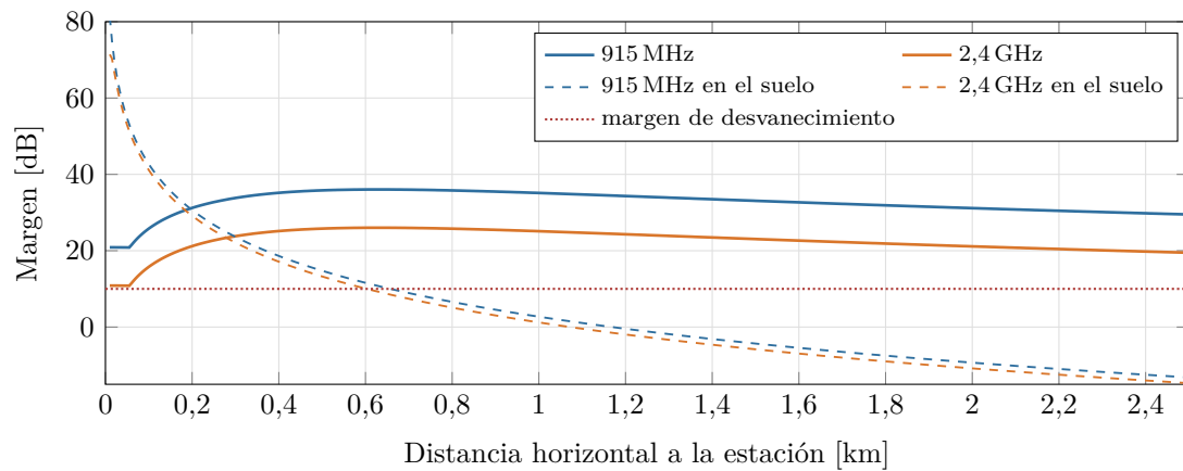
Figura 14.5: Margen del enlace con el CanSat a 560 m (Friis y diagrama del dipolo) y ya aterrizado, con la antena a 0,3 m del suelo (dos rayos con reflexión -1 , antena de tierra a 1,5 m). La caída cerca de 0 es el nulo del dipolo sobre la estación.
