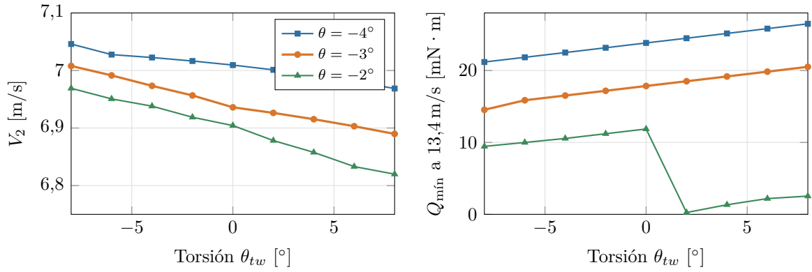
Figura 8.7: Efecto de la torsión lineal (paso referido a 0,75R ; \theta_{tw} > 0 sube el paso de la punta). A la derecha, el par mínimo de Q(\Omega) entre 0 y el equilibrio durante el arranque a 13,4\text{ m/s} .
