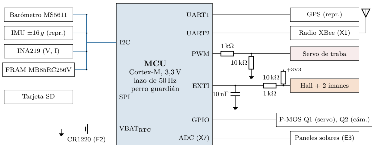
(b) Señales: buses, entradas con acondicionamiento y salidas.
