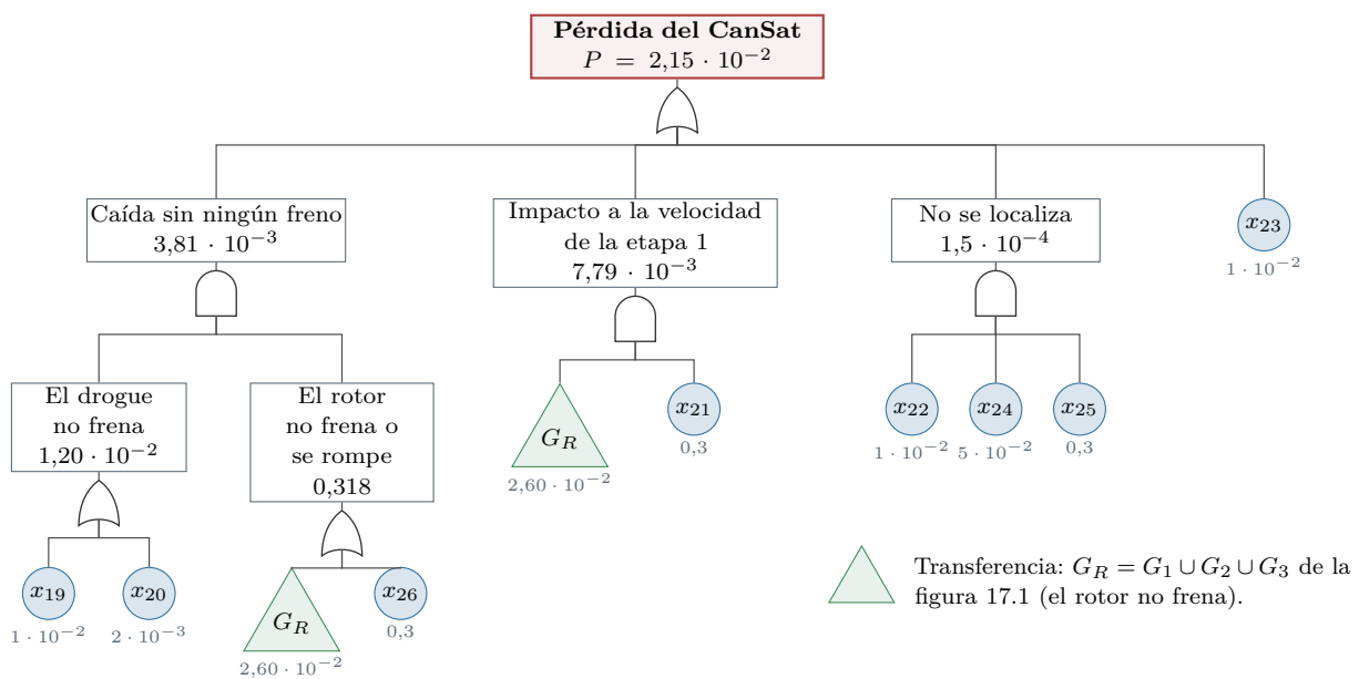
Figura 17.2: Árbol de fallas del evento “pérdida del CanSat”. x_{21} , x_{25} y x_{26} son probabilidades condicionales.
