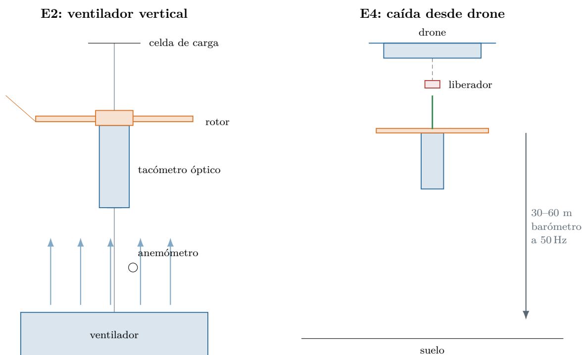
Figura 15.1: Esquemas de los ensayos E2 y E4.
