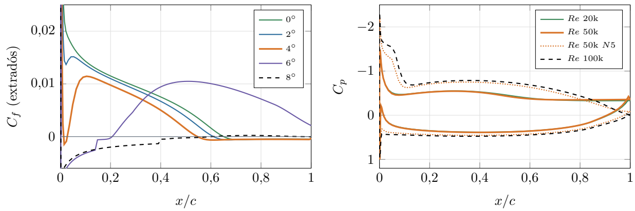
Figura 7.8: Izquierda: coeficiente de fricción del extradós de la placa al 7 % a Re = 50\,000 ( C_f < 0 : flujo separado). Derecha: distribución de presión a \alpha = 4^\circ para varios Re y N_{crit} .
