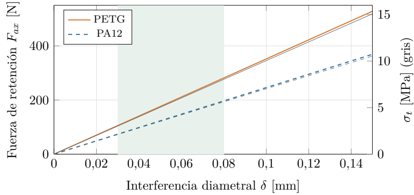
Figura 12.3: Ajuste a presión del 688ZZ en el cubo impreso, ecuación (12.9) con D_o = 30 mm. Banda verde: interferencia adoptada. Los valores no incluyen la relajación del plástico.
