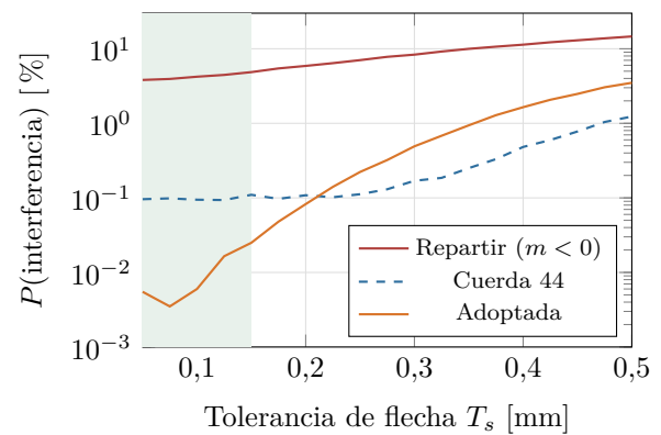
(b) Probabilidad de que una pala salga de Ø 95 o toque el cuerpo.
