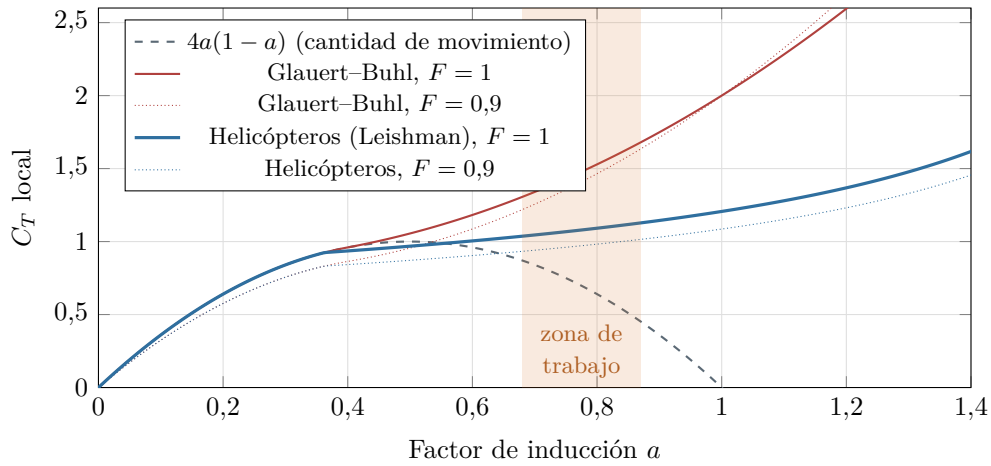
Figura 8.1: Cierres de cantidad de movimiento en el estado de molino turbulento. La banda naranja marca el intervalo de a en que trabajan los anillos del rotor en el punto de diseño.
