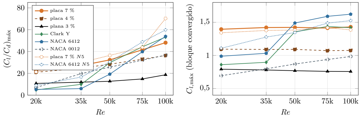
Figura 7.6: Eficiencia máxima y C_{l,\text{máx}} en función de Re . Línea llena: N_{\text{crit}} = 9 ; punteada con marcas huecas: N_{\text{crit}} = 5 .
