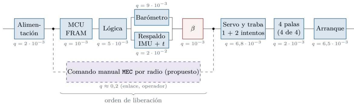
Figura 17.5: Diagrama de bloques de la cadena de liberación (configuración D, más el comando manual propuesto de la configuración E). q : probabilidad de falla por vuelo de cada bloque.
