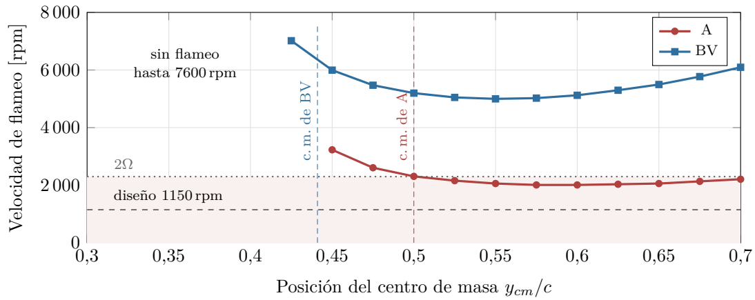
Figura 9.3: Velocidad de flameo de la sección típica en función de la posición del centro de masa (sin flameo hasta 7600 rpm: punto ausente). Con el centro de masa por delante de \approx 0,43c (A) o de \approx 0,41c (BV) no hay flameo en ese rango.
