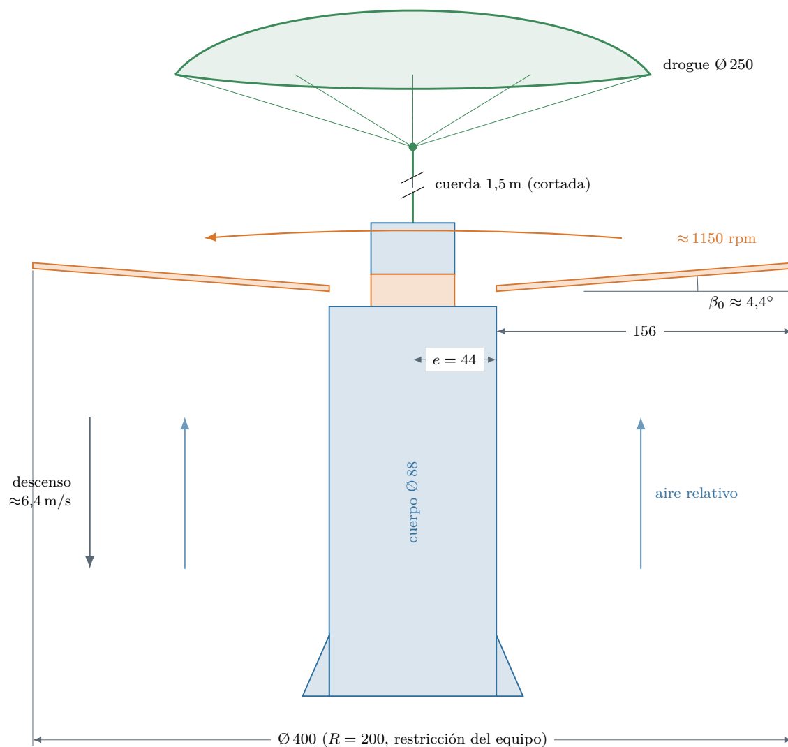
Figura 10.2: Plano 2a: conjunto desplegado, vista lateral (escala aproximada 1:3). La cuerda del drogue está cortada; su largo real es 1,5 m.
