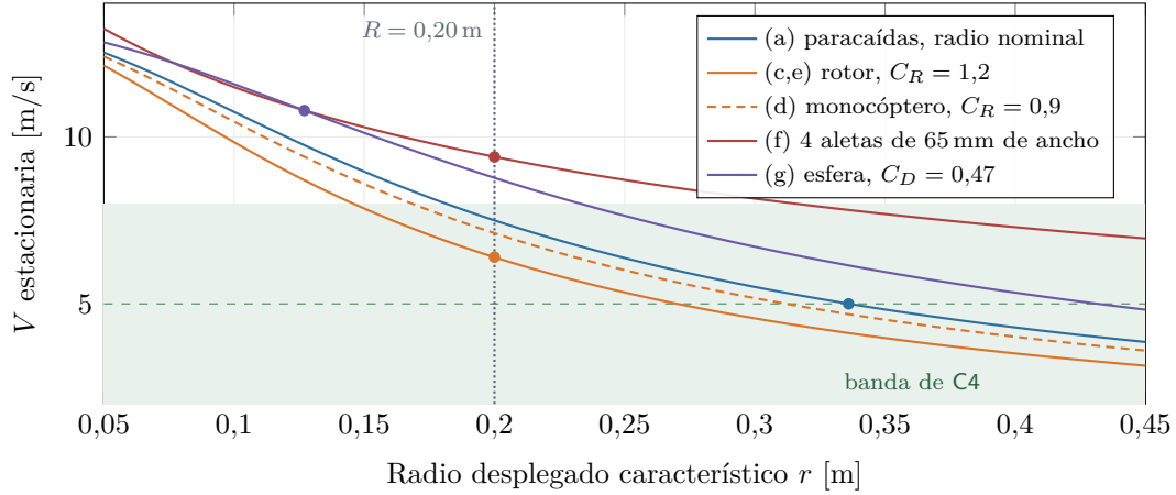
Figura 18.1: Velocidad de descenso frente al tamaño radial desplegado, con el drogue aportando por completo ( f = 1 ). Los puntos marcan el diseño de cada alternativa: el paracaídas de \varnothing 0,67 m nominal, el rotor de R = 0,20 m, las aletas de 152 mm y la esfera que infla un cartucho de 16 g de \text{CO}_2 . Para el paracaídas, r es el radio nominal (tela extendida); inflado, su radio proyectado es unos dos tercios de ese valor. Datos: decision_alternativas.py .
