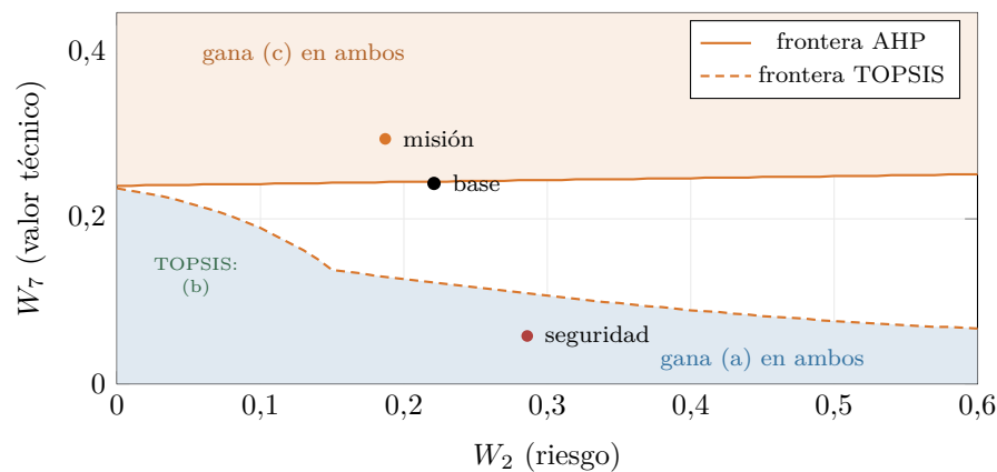
Figura 18.8: Frontera para caídas/autogiro en el plano riesgo-valor técnico (los otros cinco pesos conservan sus proporciones base; los puntos de los escenarios, que no cumplen esa condición, se ubican de forma aproximada). Entre las dos curvas los métodos discrepan. En el AHP gana siempre (a) o (c); en TOPSIS, bajo su curva, gana (a), salvo en la esquina de riesgo bajo ( W_2 \lesssim 0,15 , W_7 \approx 0,05\text{--}0,2 ), donde gana el paracaídas.
