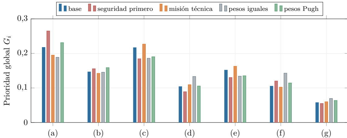
Figura 18.4: Prioridades globales del AHP en cinco escenarios de pesos.
