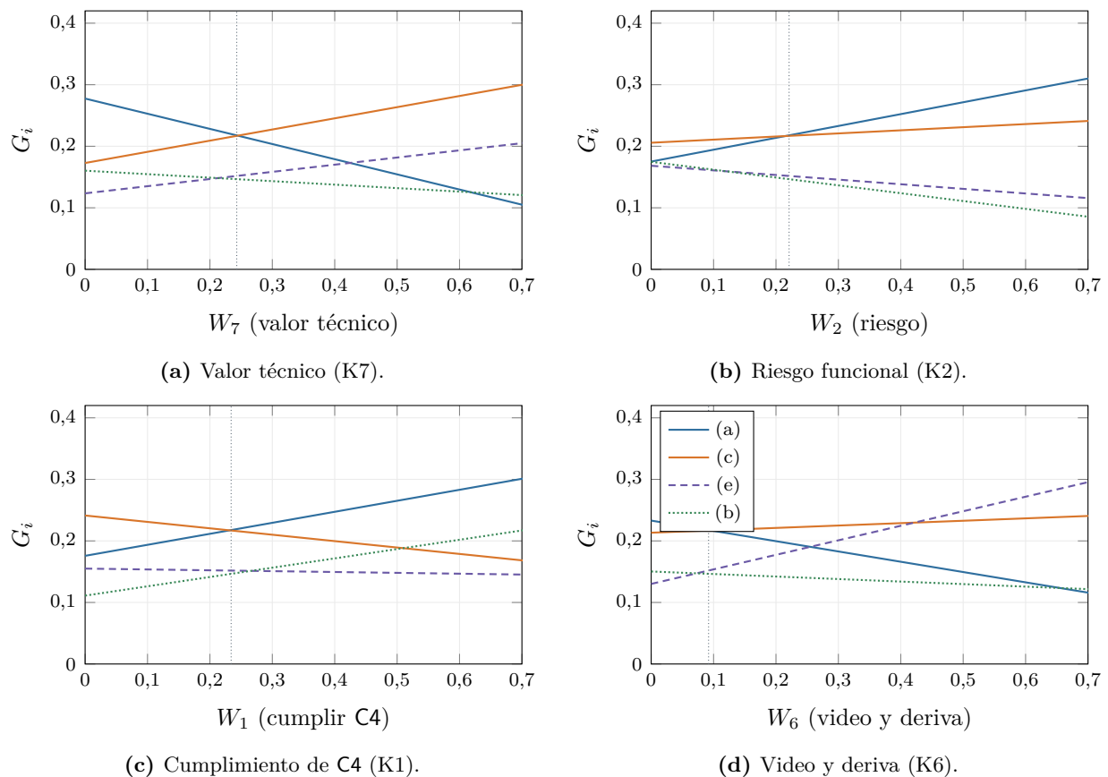
Figura 18.6: Prioridad global del AHP al variar un peso (los demás se reescalan en proporción). La línea punteada vertical marca el peso base. Azul: paracaídas; naranja: autogiro; violeta: coaxial; verde: parapente.
