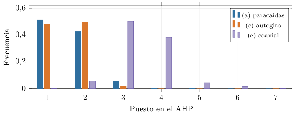
Figura 18.5: Distribución del puesto de (a), (c) y (e) en el AHP con pesos Dir( 30 \mathbf{W}_0 ). El autogiro queda primero o segundo en el 98 % de los casos.
