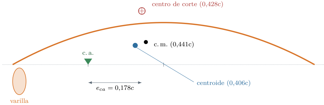
Figura 9.1: Sección de la pala (escala horizontal \approx 2,9:1 ; escala vertical exagerada al doble de la horizontal, por eso la varilla se ve como un óvalo). El centro de corte de la placa sola cae en el 50 % de la cuerda, por encima del arco; el centro aerodinámico (c. a.), en el 25 %. La varilla del borde de ataque adelanta el centro de corte y el centro de masa.
