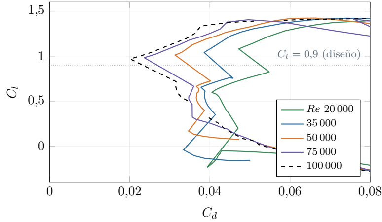
Figura 7.4: Polar C_l - C_d de la placa al 7%. La línea de puntos marca el C_l de diseño usado para estimar las rpm (ec. 5.11).
