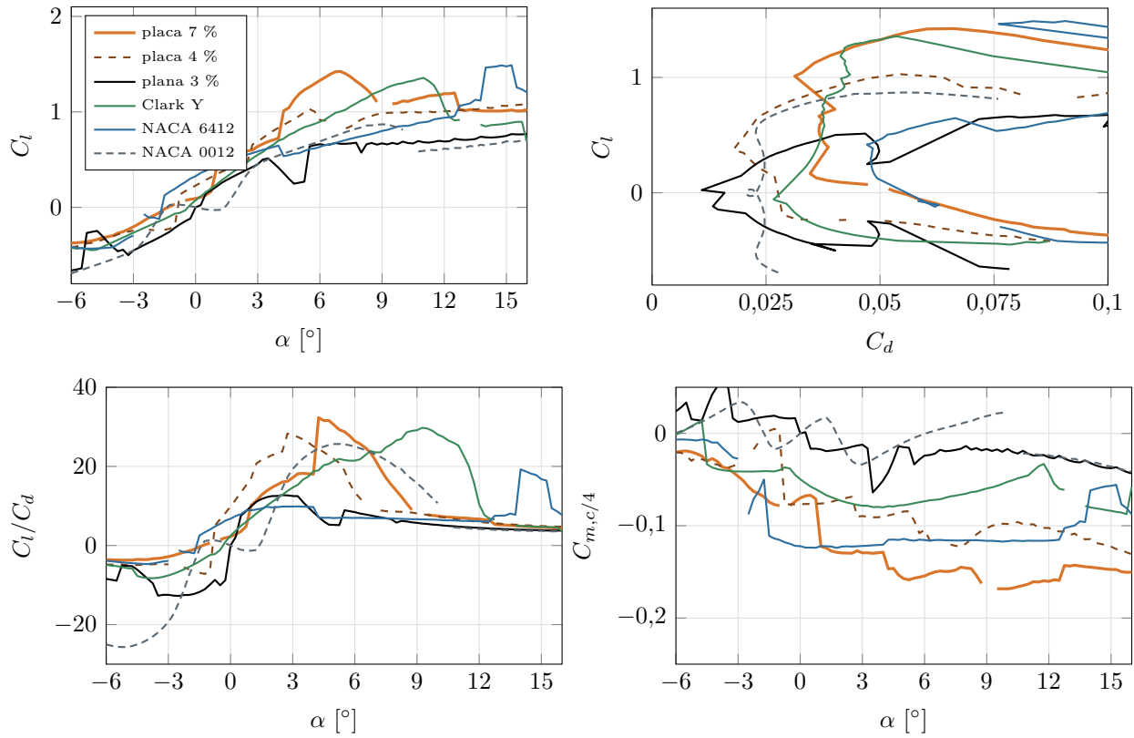
Figura 7.5: Comparación de las seis secciones a Re = 50\,000 , N_{crit} = 9 .
