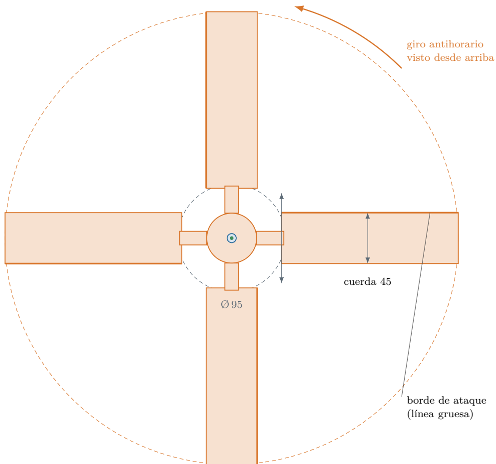
Figura 10.3: Plano 2b: rotor desplegado, planta (escala aproximada 1:3,5). La línea gruesa de cada pala es el borde de ataque.
