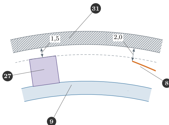
Detalle X (sección A-A), 3:1
