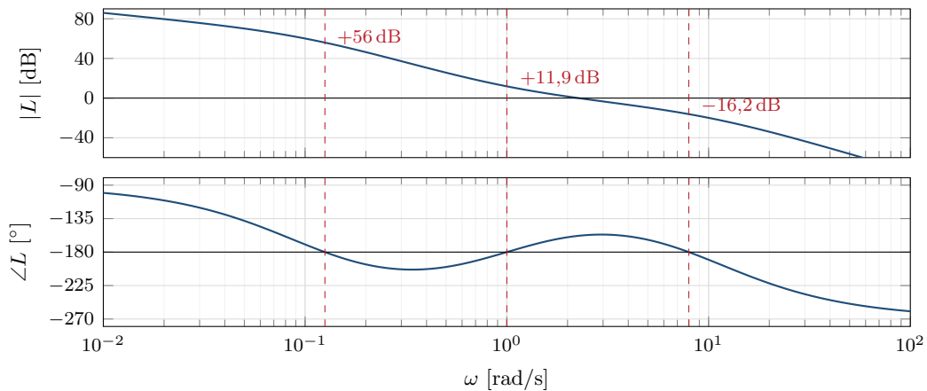
Figura 6: Lazo condicionalmente estable con K = 200 . La fase cruza -180^\circ tres veces (líneas rojas). En los dos primeros cruces |L| > 0 dB, y aun así el lazo es estable porque sus rodeos se cancelan. El margen del segundo cruce es de reducción de ganancia.
