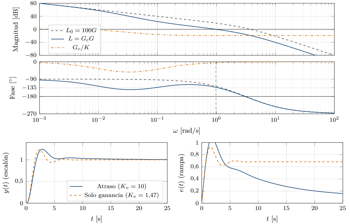
Figura 13: Ejemplo 4. Arriba: el atraso baja la curva 19 dB sin tocar la baja frecuencia. El lazo cruza en \approx 1 rad/s, donde todavía hay fase. Abajo: escalón y error ante rampa contra el ajuste por ganancia sola.
