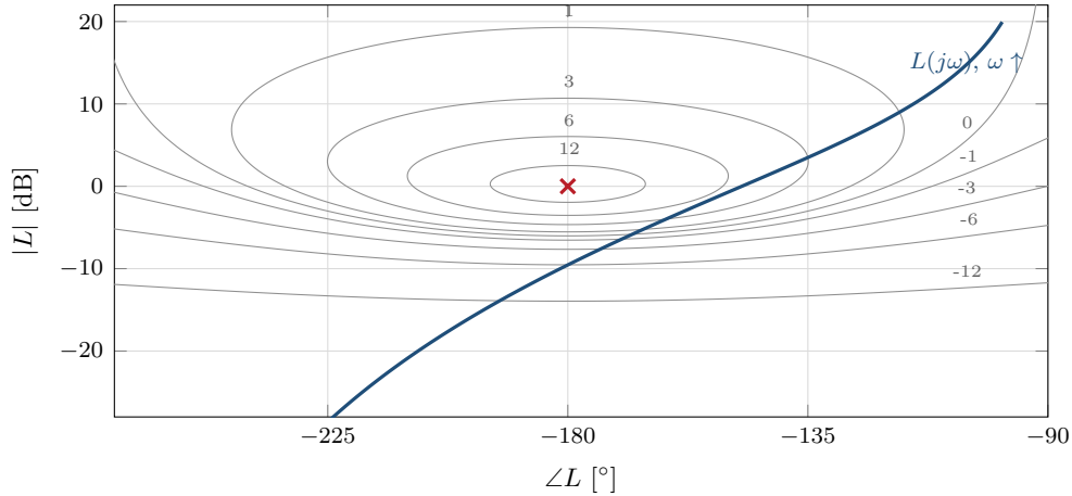
Figura 7: Carta de Nichols con L = 2/[s(s+1)(s+2)] . Los contornos grises son |T| constante en dB. La curva queda tangente a un contorno intermedio entre los de 3 y 6 dB: M_r = 5,3 \text{ dB} en \omega_r = 0,82 \text{ rad/s} , coherente con su MF = 32,6^\circ .
