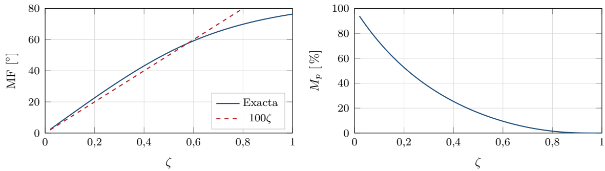
Figura 8: Margen de fase y sobrepico en función de \zeta para el segundo orden estándar.
