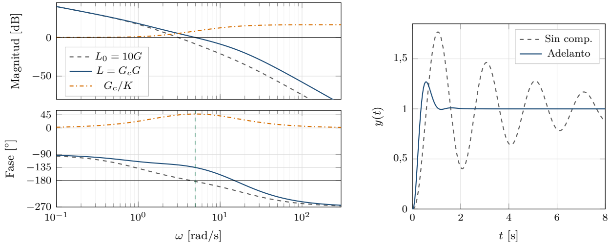
Figura 11: Ejemplo 3. Izquierda: el adelanto suma fase justo en el nuevo cruce (línea verde). Derecha: respuesta al escalón de lazo cerrado.
