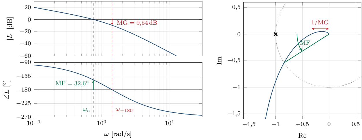
Figura 6: Márgenes de L(s) = 2/[s(s+1)(s+2)] sobre el Bode (izquierda) y sobre el diagrama polar, junto al círculo unitario (derecha).
