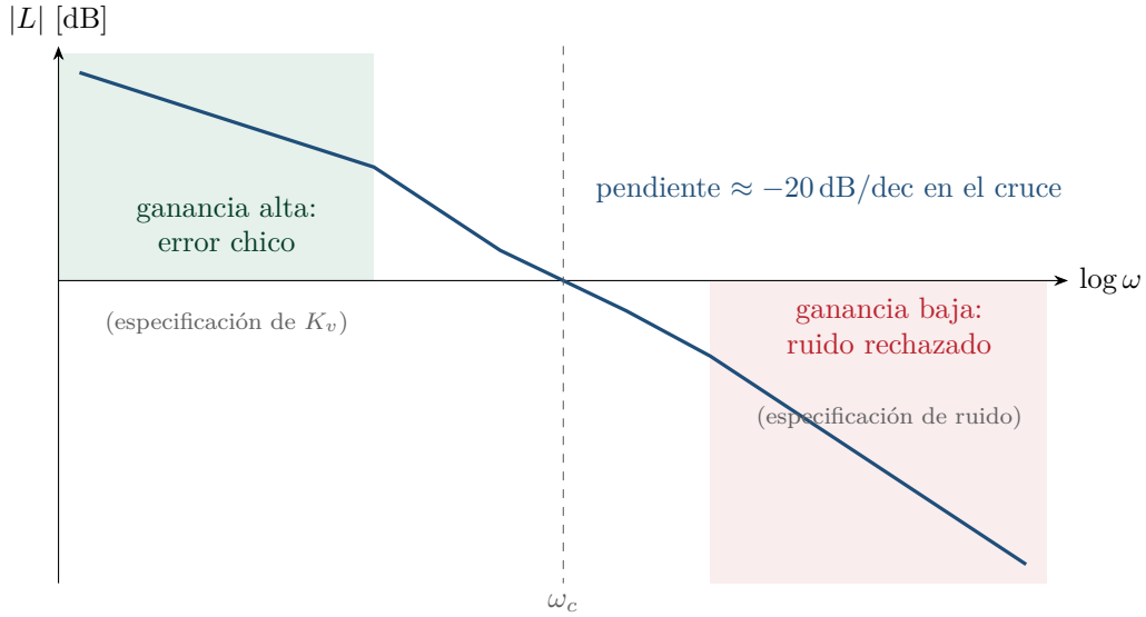
Figura 9: Esquema de la forma deseada de |L(j\omega)| . La curva debe esquivar las dos zonas sombreadas y cruzar 0 dB suavemente.
