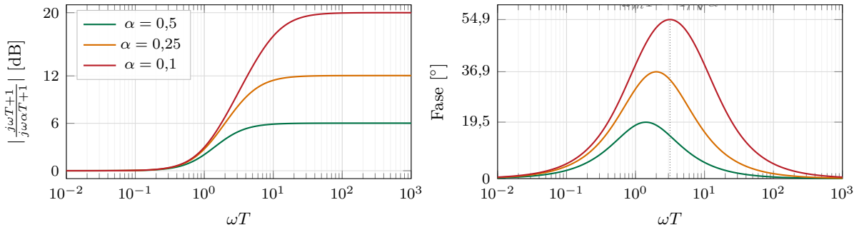
Figura 10: Red de adelanto normalizada. La fase máxima se da en la media geométrica del cero y el polo.
