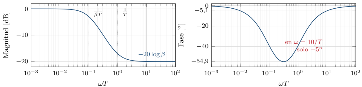
Figura 12: Red de atraso normalizada con \beta = 10 . Una década por encima del cero ya atenúa casi los 20 dB completos y atrasa apenas 5^\circ .
