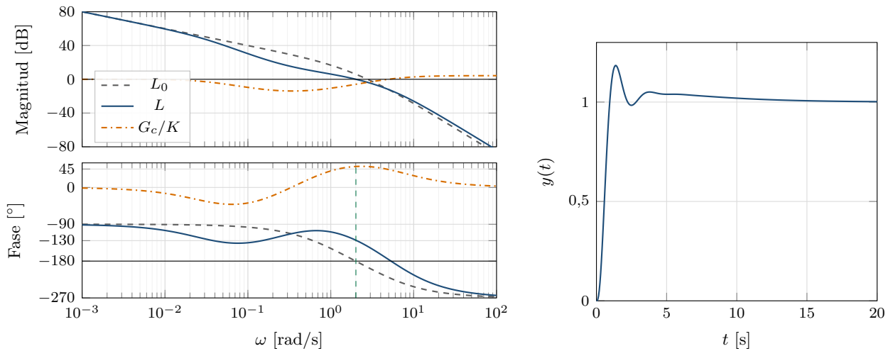
Figura 14: Ejemplo 5. La red combinada atenúa en la zona media (atraso) y suma fase alrededor de 2 \text{ rad/s} (adelanto).
