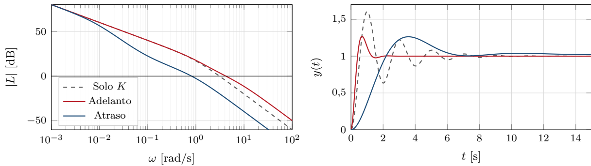
Figura 15: Adelanto contra atraso sobre G = 1/[s(s+1)] con K_v = 10 . El adelanto sube \omega_c y el atraso lo baja.
