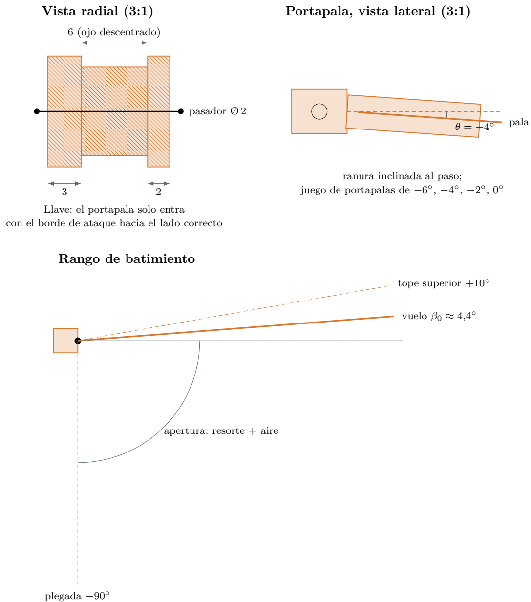
Figura 6.7: Plano 6: bisagra de batimiento. Orejas asimétricas como llave de montaje (un portapala dado vuelta no entra); paso fijado por la ranura del portapala; rango de movimiento de la pala entre plegada ( -90^\circ ) y el tope superior ( 10^\circ ).
