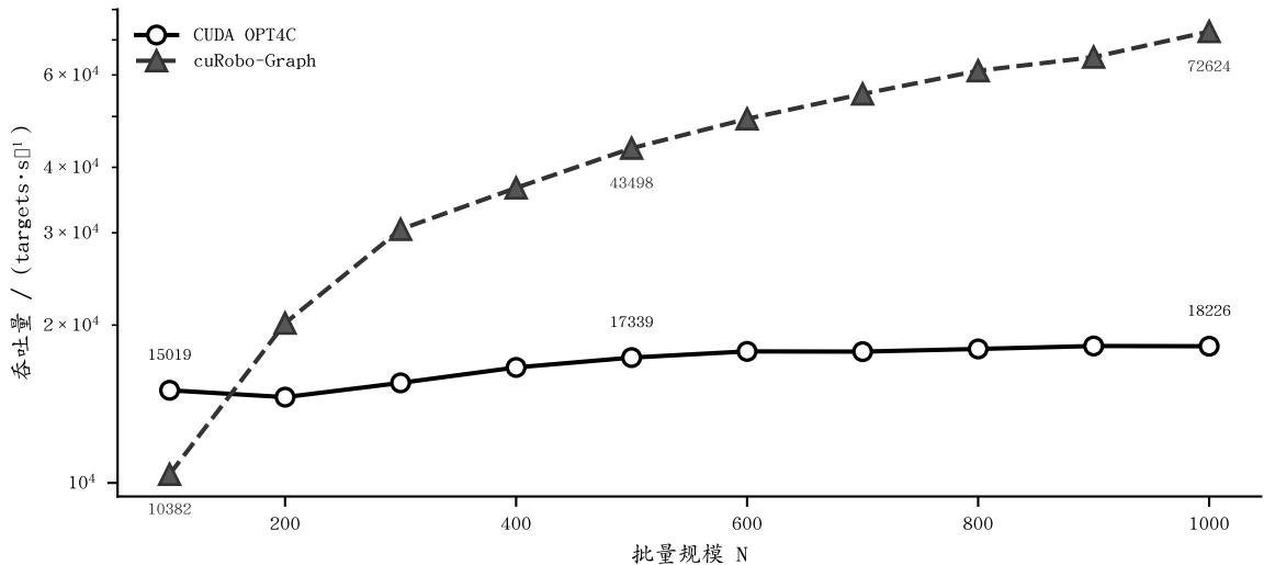
CUDA OPT4C 与 cuRobo-Graph 批量吞吐量对比
