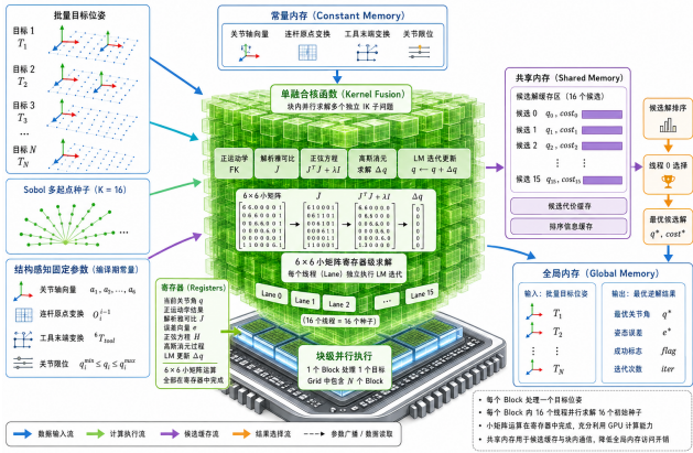
图 4 机械臂逆运动学在统一计算架构上的求解流程与数据流
