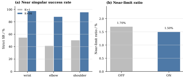
图6 近奇异与近限位场景边界分析。子图 (a) 比较 wrist、elbow 和 shoulder 近奇异目标下 K = 1 与 K = 16 的 Strict 成功率；子图 (b) 比较 Barrier ON/OFF 下的 near-limit ratio。
