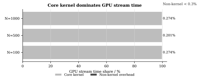
图2 OPT4C 核函数时间与非 kernel 开销组成。非 kernel 开销包含 H2D、D2H 和 launch， N = 1000 时占比低于 0.3%。
