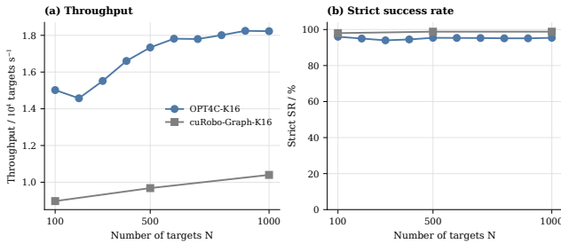
图 3 同种子数 K = 16 条件下 OPT4C 与 cuRobo-Graph 的批量吞吐率和 Strict 成功率对比。
