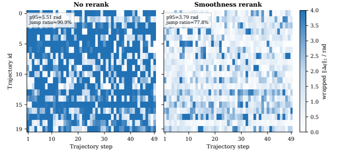
图7 轨迹相邻点关节跳变量热图。 \Delta q 采用旋转关节 wrap 差分计算, 两个子图共享 0–4 rad 色标, 并标注 p_{95} 与 jump ratio。
