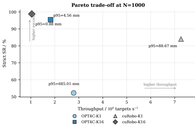
图 4 吞吐率-成功率-误差三目标关系 ( N = 1000 )
