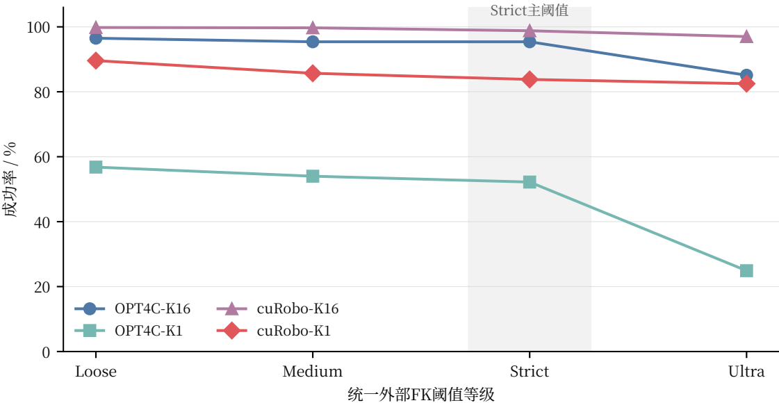
N=1000 阈值扫描：逐目标误差重算
