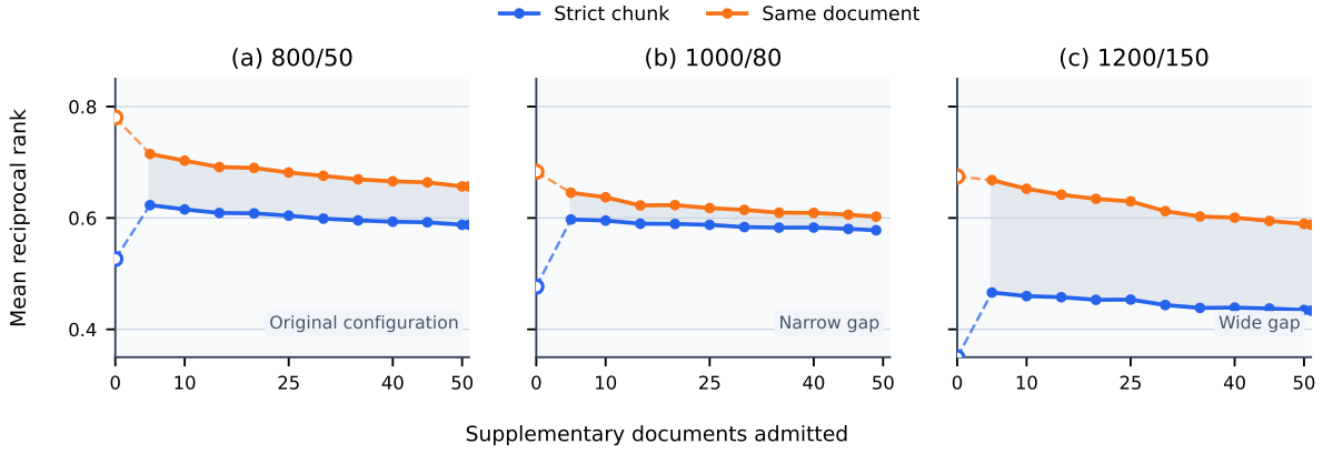
图 8: 三个代表性 nomic-embed-text 分块配置下的自检索结果。蓝线为严格同分块匹配, 橙线为同文档匹配, 阴影表示两种匹配标准的差距; 纵轴为平均倒数排名, 越高表示目标段落首次出现的位置越靠前。空心点为仅核心资料基线, 虚线只连接基线与首个扩库点, 实线比较相同扩库规模下的两种匹配标准。
