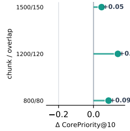
图 6：多语 MiniLM 编码器在加入 10 份补充资料时，技术细节查询相对基线查询的平均核心资料前十名占比变化。每点对应一个字符分块设置，左图纵轴标出两图共享的分块长度/重叠；正值表示技术细节查询家族的权威资料可见性较高。
