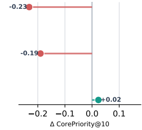
图 6：多语 MiniLM 编码器在加入 10 份补充资料时，技术细节查询相对基线查询的平均核心资料前十名占比变化。每点对应一个字符分块设置，左图纵轴标出两图共享的分块长度/重叠；正值表示技术细节查询家族的权威资料可见性较高。
