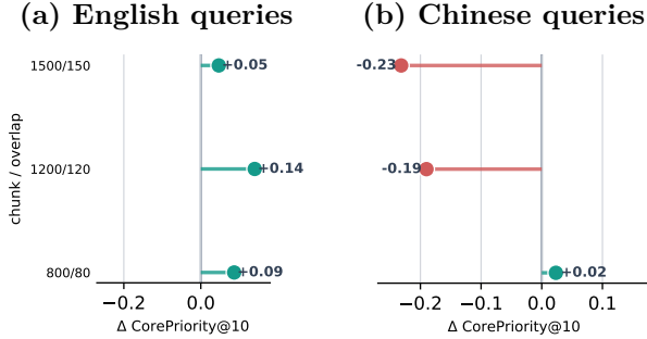
图 5: 多语 MiniLM encoder 在加入 10 份补充资料时，技术细节 query 相对基线 query 的平均 CorePriority@10 变化。每点对应一个字符分块设置，左图纵轴标出两图共享的分块长度/重叠；正值表示技术细节 query 家族的核心来源可见性 (CorePriority@10) 较高。
