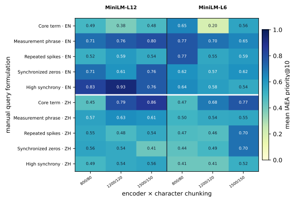
图 6: m = 10 时 query、语言、encoder 与字符分块方式的交互。每个单元格为 CorePriority@10 的平均值；横向分隔线区分英文与中文 query，纵向分隔线区分两种 encoder。由 observation packet 线索形成的技术细节 query 并不在所有语言和配置下提高核心来源可见性。
