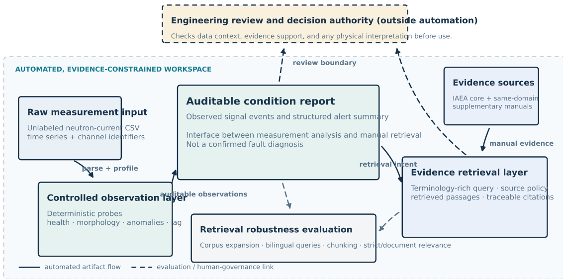
图 1: 测量—证据接口的研究总览 (V2 占位图)。原始中子电流记录经确定性分析形成可回溯观察与结构化摘要; 摘要在来源策略约束下连接至可定位的技术证据, 并组织为供工程师复核的候选解释。正式版本将按 V3 术语重绘。
