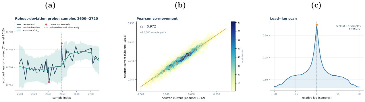
图 2: 确定性 probes 所描述的统计现象示例: (a) 样本 2600~2720 的局部稳健偏离规则, 纵轴为相应通道记录的中子电流值; (b) 通道间 Pearson 共变; (c) 相关-滞后扫描。它们用于说明 observation packet 中可保存的描述性证据, 不构成已确认故障或因果方向。
