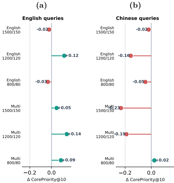
图 5: 加入 10 份补充资料时，技术细节 query 相对基线 query 的平均 CorePriority@10 变化。每点对应一个 encoder-字符分块设置；正值表示技术细节 query 家族的核心来源可见性 (CorePriority@10) 较高。(a) 英文设置；(b) 中文设置。
