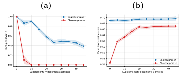
图 4：字符分块扩库下的语义相似度与核心资料在前 10 个结果中的占比（来源可见性）。结果聚合 17 个已保存分块配置；阴影表示配置间标准差。(a) CorePriority@10 可随相关补充资料加入而下降；(b) 在相同协议中，平均最高余弦相似度提高或保持稳定。两者可同时发生。
