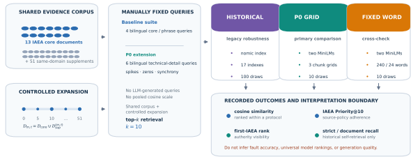
图 3: 分层评价设计与检索协议（V2 占位图）。在固定的资料库、查询集和 top-k 规则下，评价分别核查测量侧 observation packet 的可回溯性，以及资料扩展、query、语言、encoder 和分块方式对前 10 个结果中核心资料占比的影响。正式版本将按 V3 评价结构重绘。
