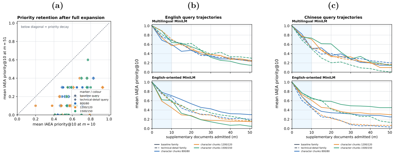
图 7: 扩库后的来源可见性保持能力: (a) 不同配置在 m=10 与 m=51 的对应关系, 落在对角线下方表示进一步衰减; (b) 英文 query 的完整扩库轨迹; (c) 中文 query 的相应轨迹。该图组展开候选配置的条件性选择, 不建立跨语言或跨 encoder 的普适排名。
