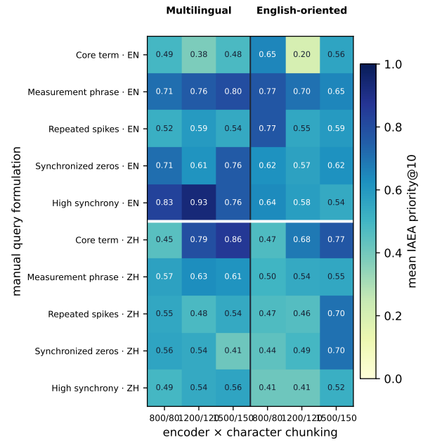
图 6: m = 10 时 query、语言、encoder 与字符分块方式的交互。每个单元格为 CorePriority@10 的平均值；横向分隔线区分英文与中文 query，纵向分隔线区分两种 encoder。由 observation packet 线索形成的技术细节 query 并不在所有语言和配置下提高核心来源可见性。
