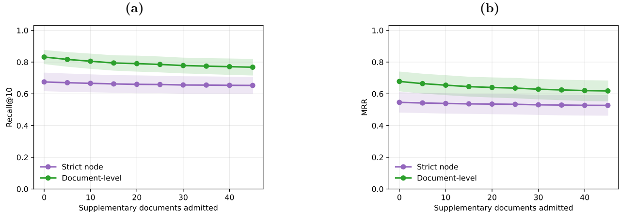
图 8: self-retrieval 的检索单元核查: (a) Recall@10; (b) MRR。两图均区分 exact-chunk 与 same-document 两种匹配标准, 用于说明重叠分块下“找回”的指标边界, 不衡量工程正确性。
