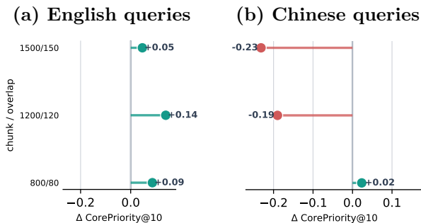
图 6: 多语 MiniLM encoder 在加入 10 份补充资料时，技术细节 query 相对基线 query 的平均 \text{CorePriority}@10 变化。每点对应一个字符分块设置，左图纵轴标出两图共享的分块长度/重叠；正值表示技术细节 query 家族的核心来源可见性 ( \text{CorePriority}@10 ) 较高。
