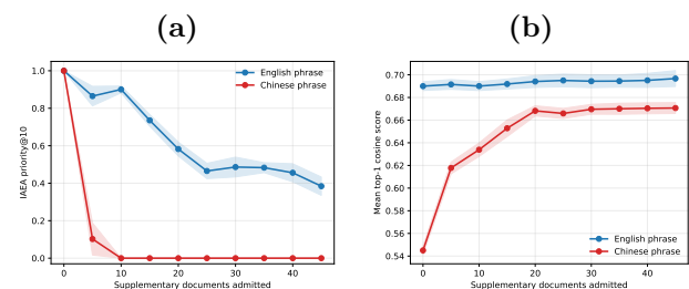
图 4：字符分块扩库下的语义相似度与核心资料在前 10 个结果中的占比（来源可见性）。结果聚合 17 个已保存分块配置；阴影表示配置间标准差。(a) CorePriority@10 可随相关补充资料加入而下降；(b) 在相同协议中，平均最高余弦相似度提高或保持稳定。两者可同时发生。
