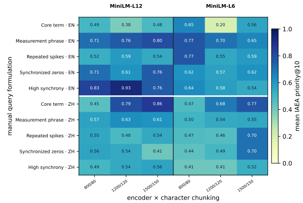
图 7: m = 10 时 query、语言、encoder 与字符分块方式的交互。每个单元格为 \text{CorePriority}@10 的平均值；横向分隔线区分英文与中文 query，纵向分隔线区分两种 encoder。由 observation packet 线索形成的技术细节 query 并不在所有语言和配置下提高核心来源可见性。
