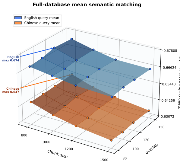
图 5: 全数据库条件下 nomic-embed-text 的中英文平均语义匹配程度。每个曲面为同一语言两条固定 query 的平均值；横轴为分块长度，纵轴为重叠长度，高度为前 10 个结果的平均余弦相似度。箭头标出各语言的最高点。
