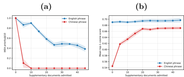
图 4：字符分块扩库下的语义相似度与核心资料在前 10 个结果中的占比（来源可见性）。结果聚合 17 个已保存分块配置；阴影表示配置间标准差。(a) 核心资料前十名占比可随相关补充资料加入而下降；(b) 在相同协议中，平均最高余弦相似度提高或保持稳定。两者可同时发生。
