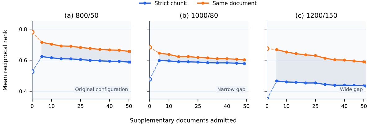
图 8: 三个代表性 nomic-embed-text 分块配置下的自检索结果。蓝线为严格同分块匹配, 橙线为同文档匹配, 阴影表示两种匹配标准的差距; 纵轴为平均倒数排名, 越高表示目标段落首次出现的位置越靠前。空心点为仅核心资料基线, 虚线只连接基线与首个扩库点, 实线比较相同扩库规模下的两种匹配标准。
