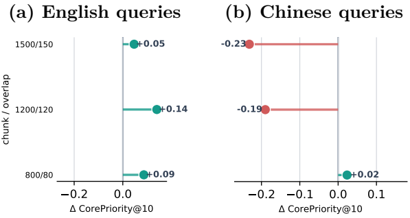
图 6: 多语 MiniLM 编码器在加入 10 份补充资料时，技术细节查询相对基线查询的平均核心资料前十名占比变化。每点对应一个字符分块设置，左图纵轴标出两图共享的分块长度/重叠；正值表示技术细节查询家族的核心来源可见性较高。
