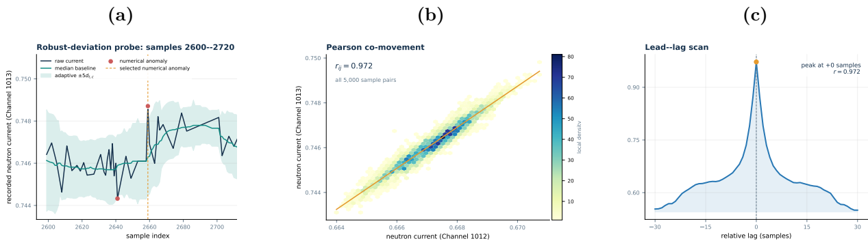
图 2: 确定性分析工具所描述的统计现象示例: (a) 样本 2600-2720 的局部稳健偏离规则, 纵轴为相应通道记录的中子电流值; (b) 通道间皮尔逊相关; (c) 相关-滞后扫描。它们用于说明观测包中可保存的描述性证据, 不构成已确认故障或因果方向。
