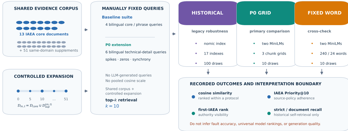
图 4.1: 分层评价设计与检索协议 (V2 占位图)。在固定的资料库、查询集和 top- k 规则下，评价分别核查测量侧 observation packet 的可回溯性，以及资料扩展、query、语言、encoder 和分块方式对核心来源可见性的影响。正式版本将按 V3 评价结构重绘。
