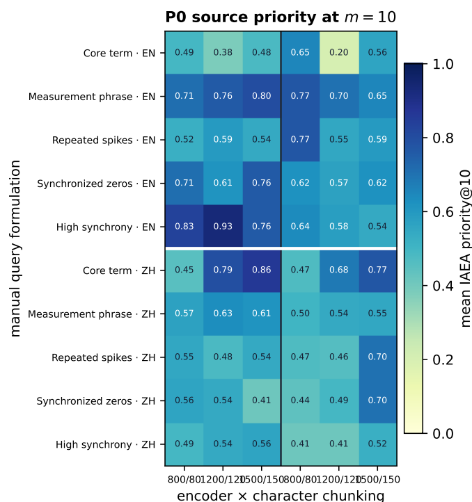
图 5.3: 不同 query 与 encoder—分块配置下的核心来源可见性 (V2 占位图, m = 10 )。该图显示 query 表述的作用随语言与配置而改变。正式版本将减少 query 行数, 并以中文标签呈现。
