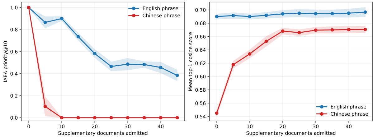
图 5.2: 资料扩展下的核心来源可见性与最高余弦相似度 (V2 占位图)。结果聚合 17 个已保存分块配置; 阴影表示配置间标准差。核心来源可见性可以下降, 即使最高余弦相似度上升或保持稳定。正式版本将统一为 V3 的中文术语与版式。
