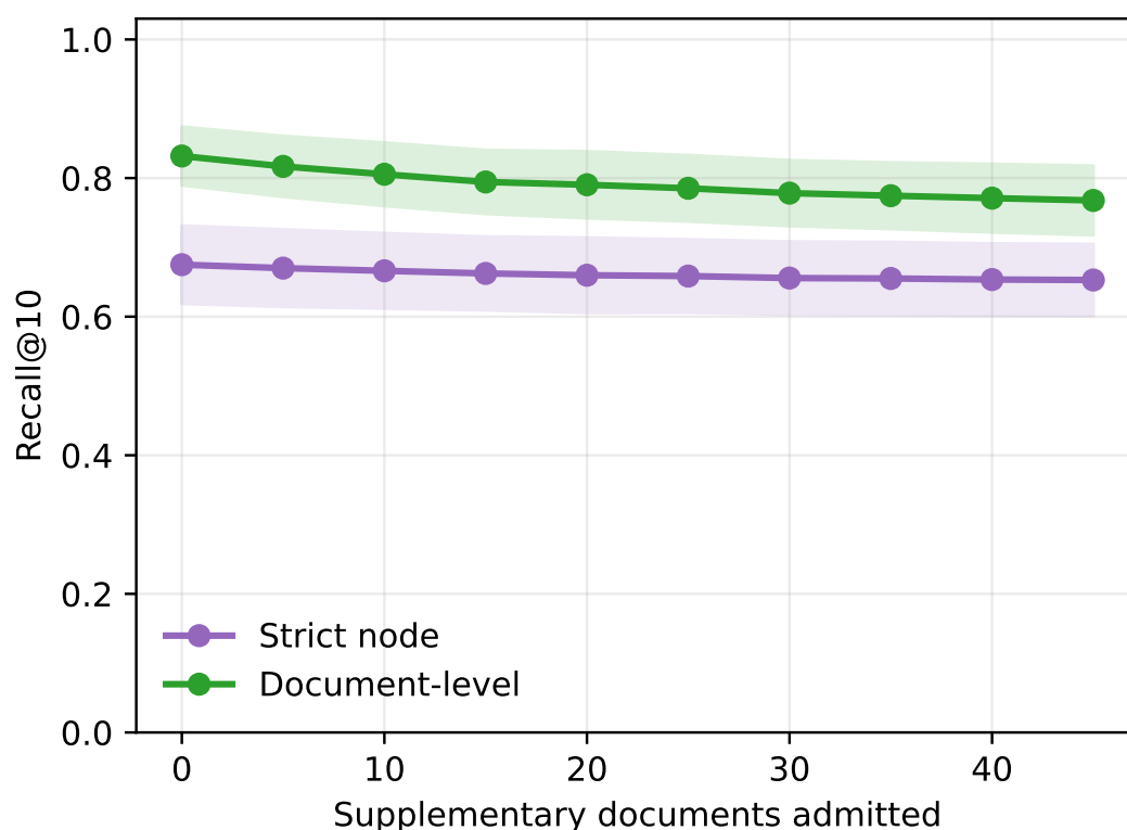
图 5.4: self-retrieval 的 Recall@10 结果 (V2 占位图)。该核查区分 exact-chunk 与 same-document 两种匹配标准, 用于解释重叠分块下检索单元与段落定位的关系, 而不衡量工程正确性。正式版本可与 MRR 合并重绘, 或移至补充材料。
