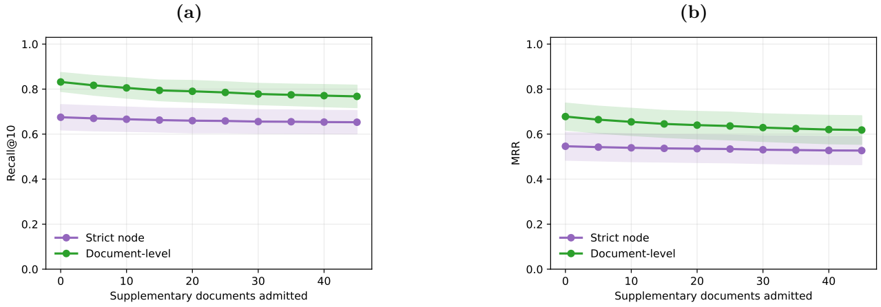
图 8: 自检索的检索单元核查: (a) 前十名召回率; (b) 平均倒数排名。两图均区分严格同分块与同文档两种匹配标准, 用于说明重叠分块下“找回”的指标边界, 不衡量工程正确性。
