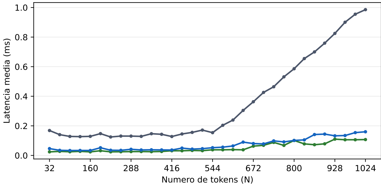
PyTorch eager PyTorch SDPA Triton custom Latencia da atencao densa
