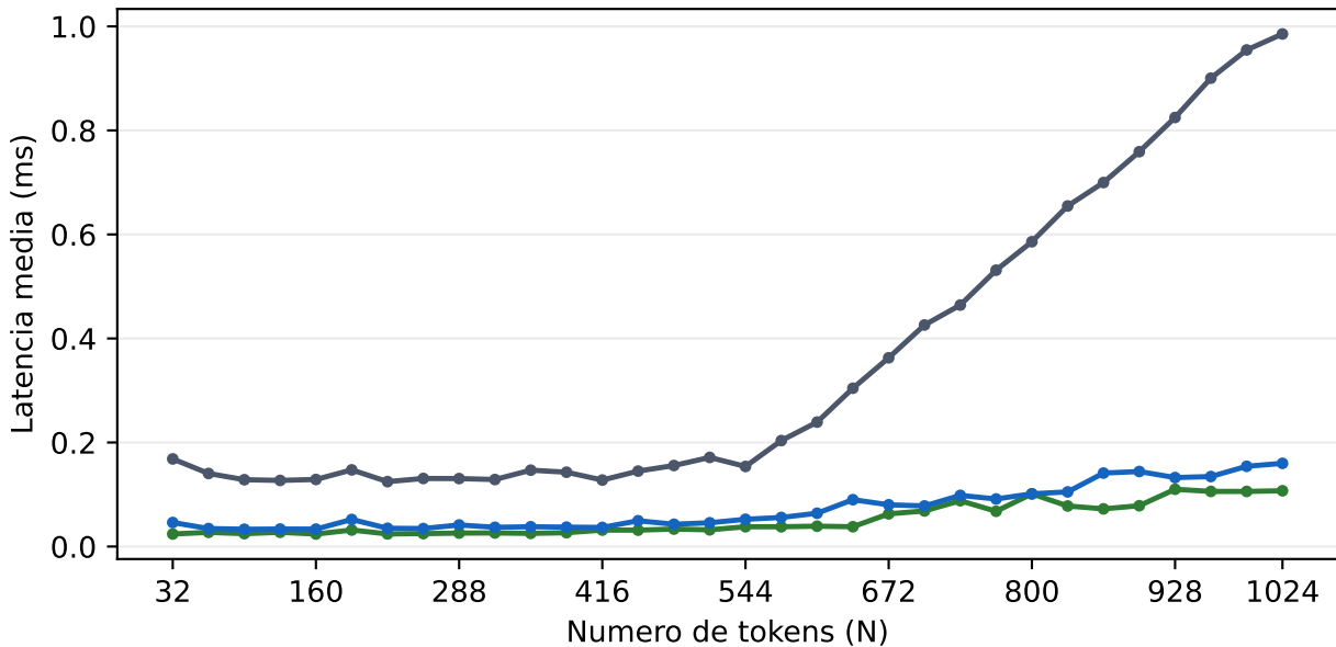
PyTorch eager PyTorch SDPA Triton custom Latencia da atencao densa
