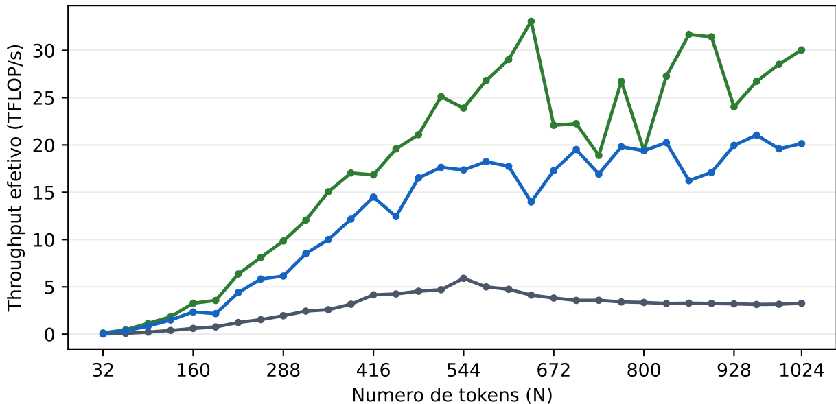
PyTorch eager PyTorch SDPA Triton custom Throughput efetivo da atencao densa
