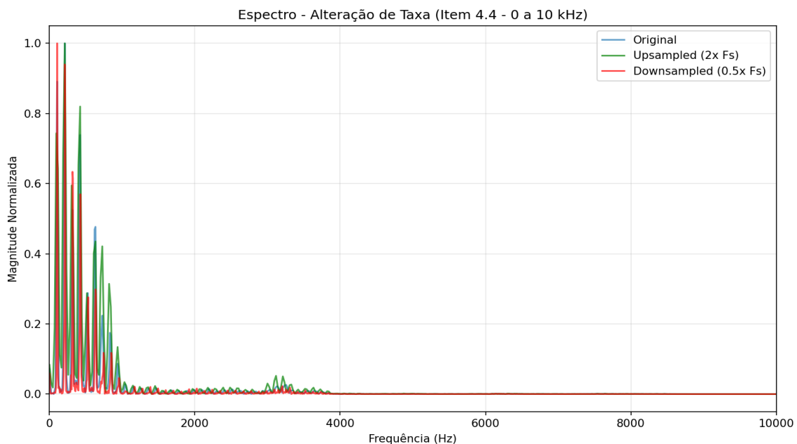
Figura 5a: Espectro da Alteração de Taxa na faixa ampla de 0 a 10 kHz.
