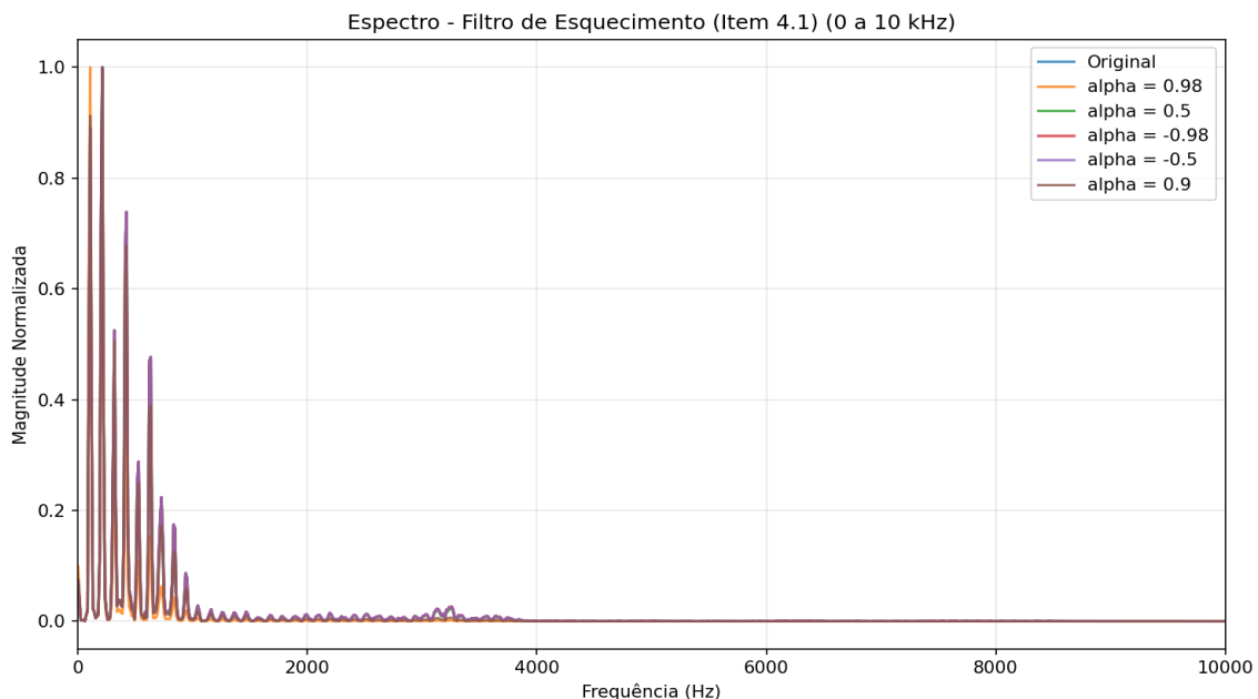
Figura 2a: Espectro do Filtro de Esquecimento na faixa ampla de 0 a 10 kHz.
