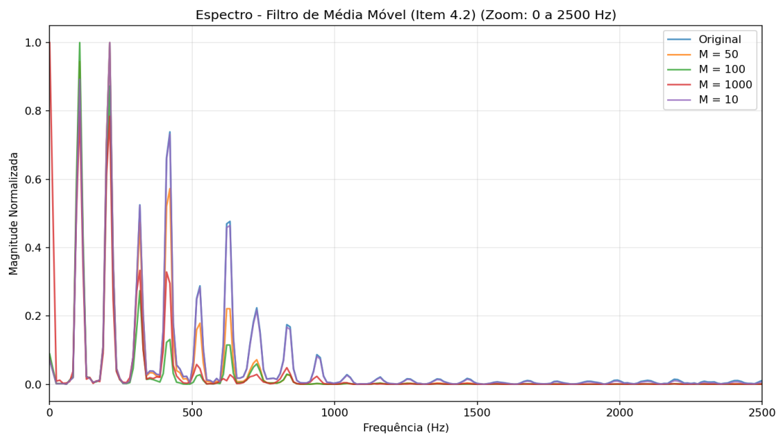
Figura 3b: Espectro do Filtro de Média Móvel com detalhamento dos formantes (Zoom: 0 a 2500 Hz).
