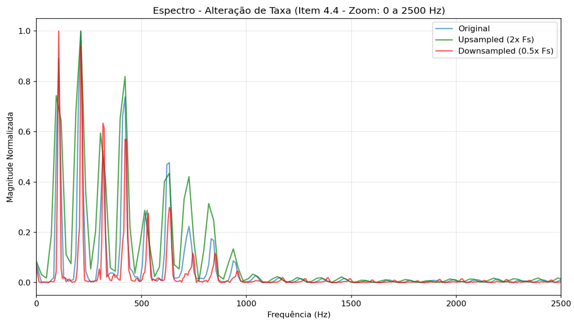
Figura 5b: Espectro da Alteração de Taxa com detalhamento dos formantes (Zoom: 0 a 2500 Hz).
