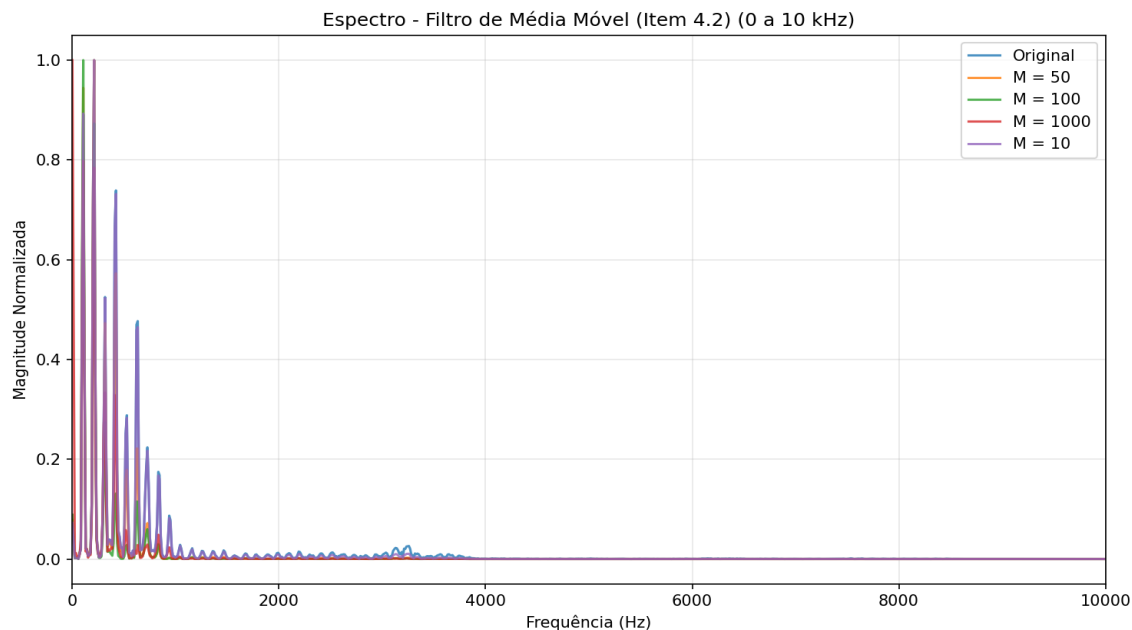
Figura 3a: Espectro do Filtro de Média Móvel na faixa ampla de 0 a 10 kHz.
