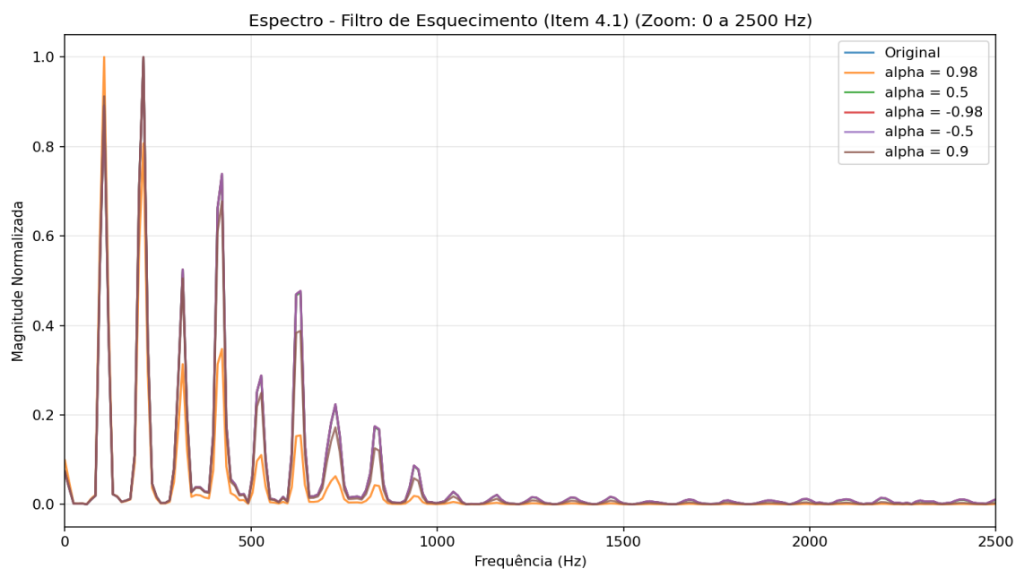
Figura 2b: Espectro do Filtro de Esquecimento com detalhamento dos formantes (Zoom: 0 a 2500 Hz).
