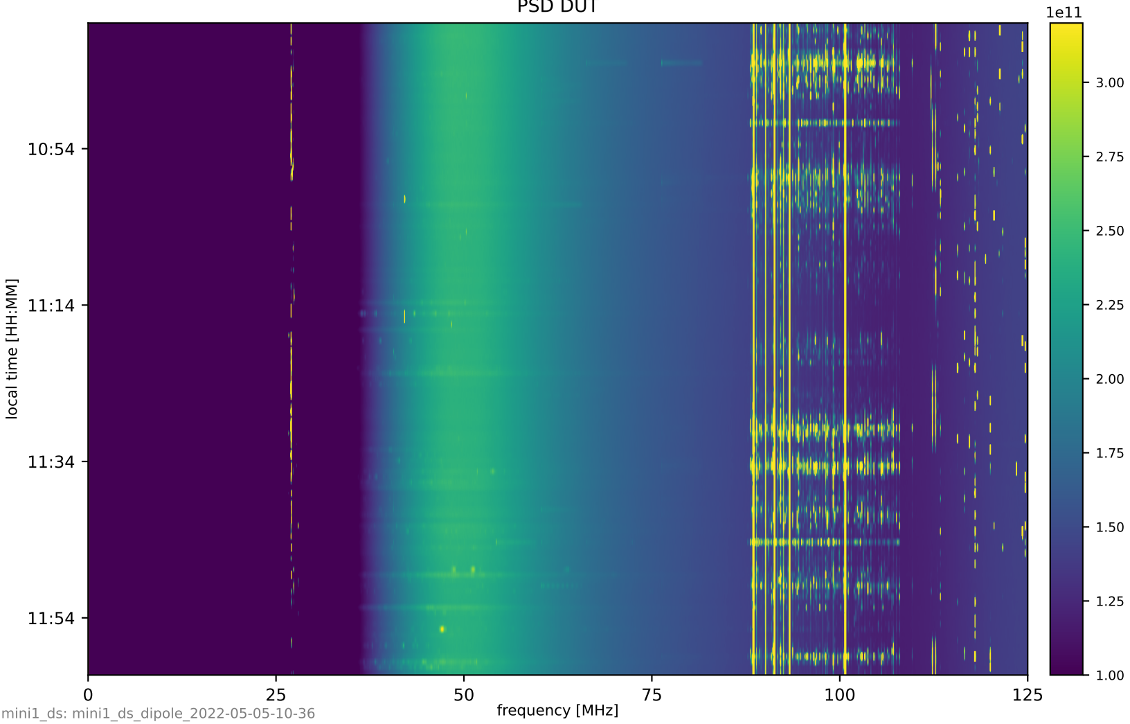
PSD DUT
