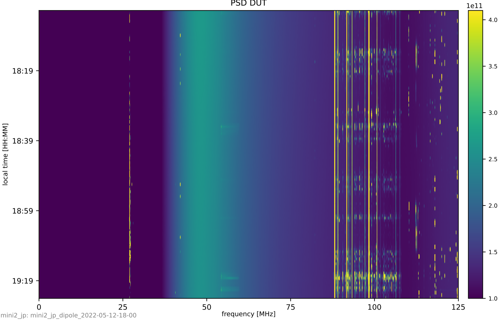
PSD DUT
