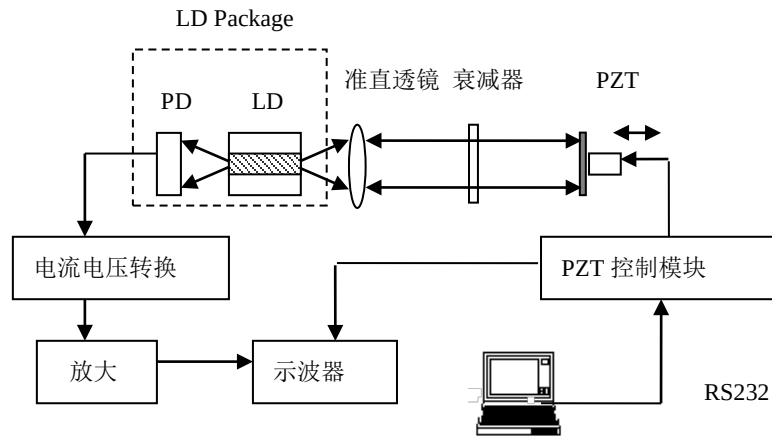
图 2.8 半导体激光自混合干涉定量观察实验系统
