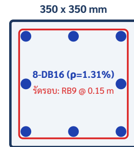
รูปตัดเสา คสล. C1 (ชั้น 1)
