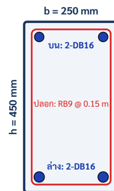
รูปตัดคาน คสล. มาตรฐาน B1 / AS1
