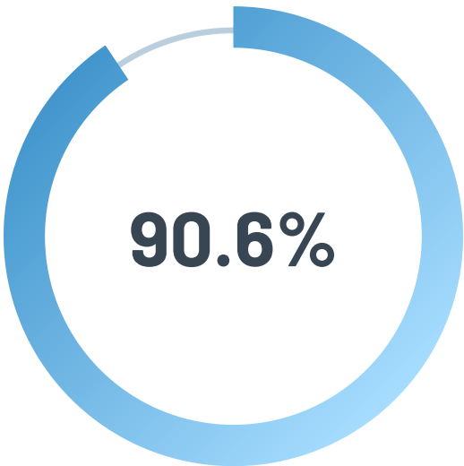
ROC-AUC
