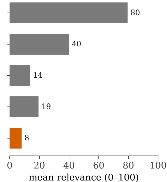
GPT-5.6
