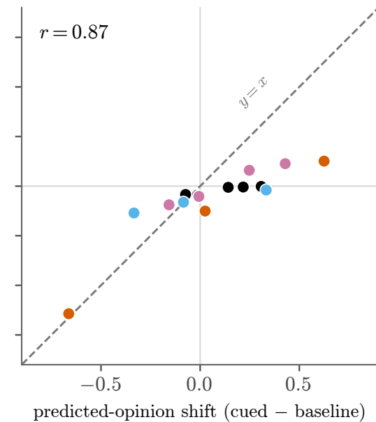
Claude Sonnet 5
