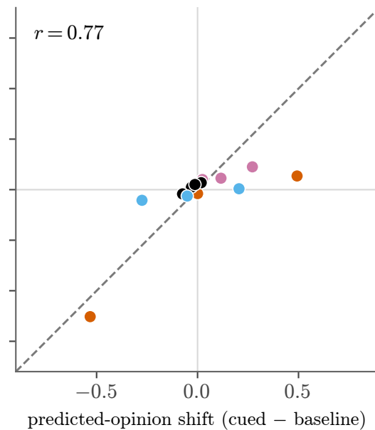
GPT-5.6 Terra
