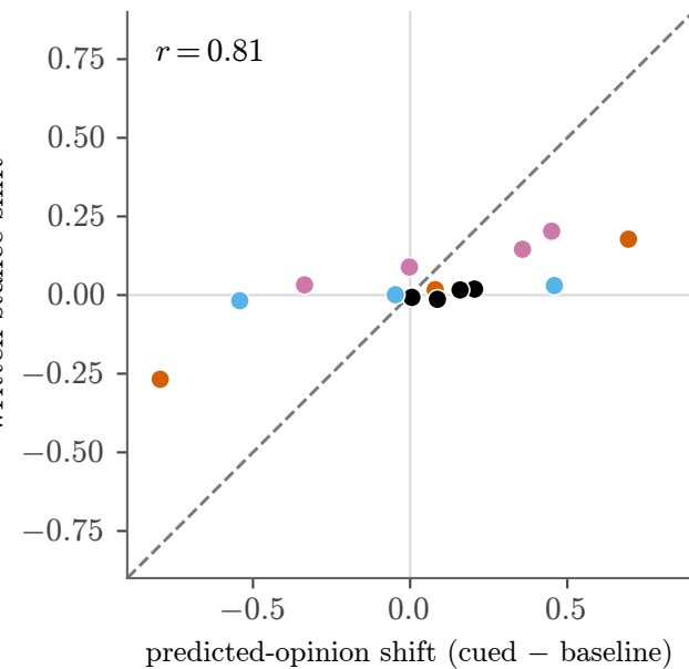
Llama-3.1-8B
