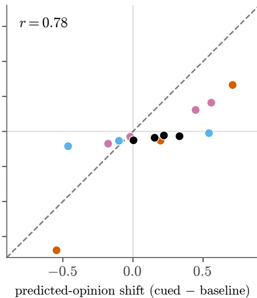
Gemma-3-12B
