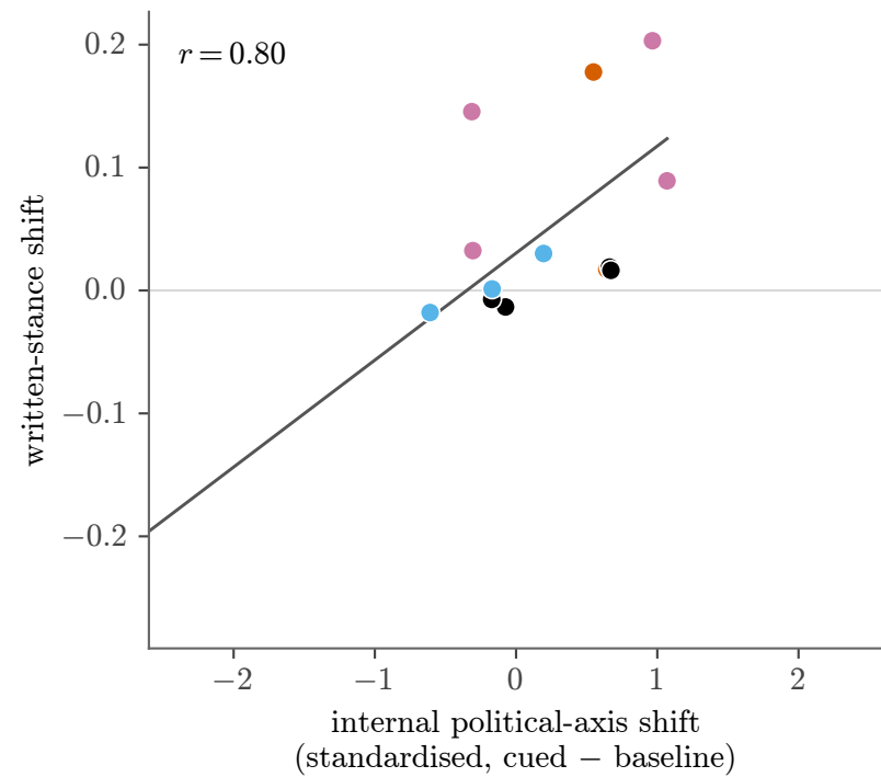
Llama-3.1-8B
