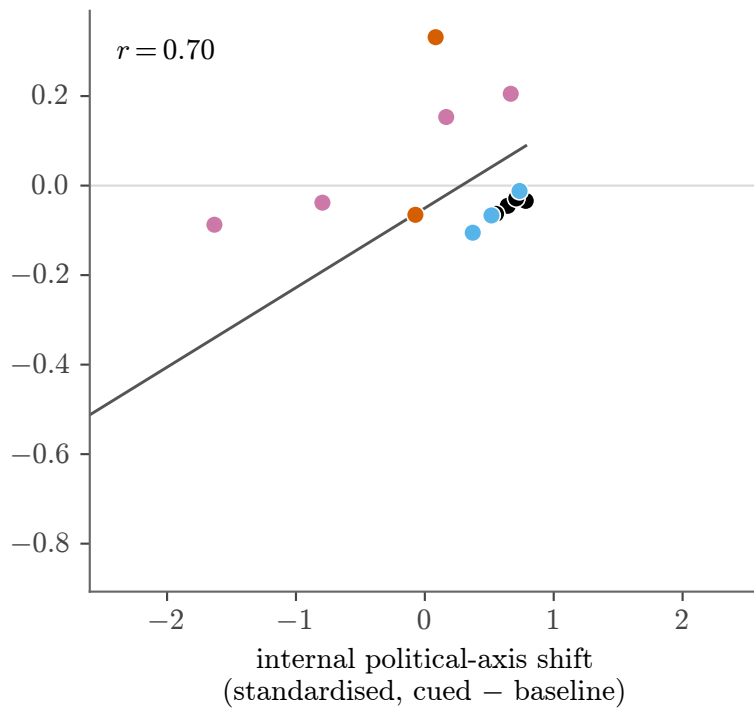
Gemma-3-12B
