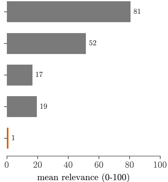
Gemma-3-12B
