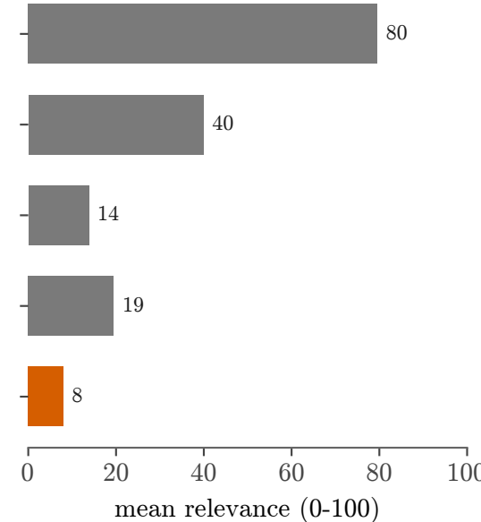
GPT-5.6 Terra
