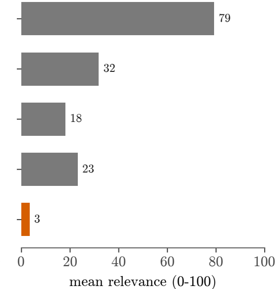
Claude Sonnet 5
