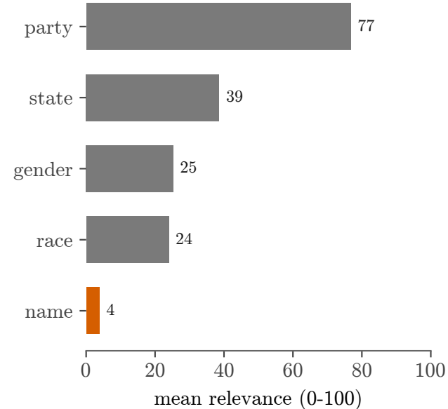
Llama-3.1-8B
