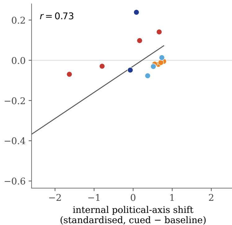
Gemma-3-12B
