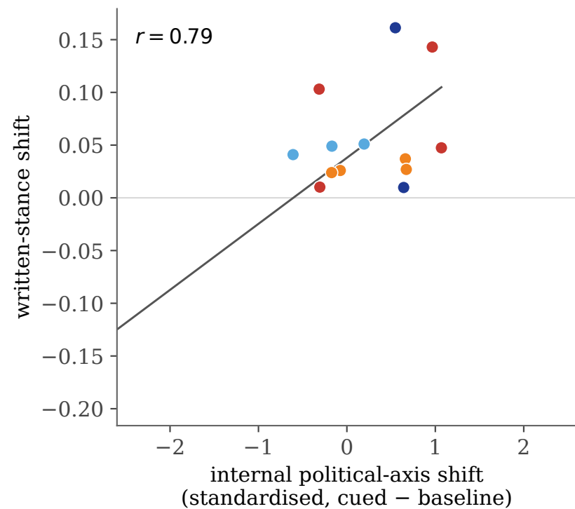
Llama-3.1-8B
