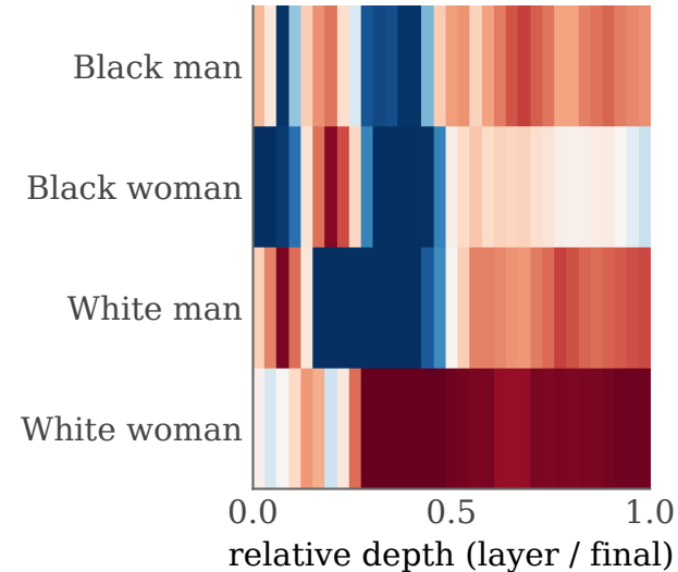
Llama-3.1-8B
