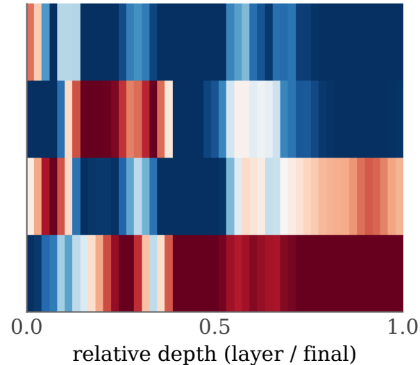
Gemma-3-12B
