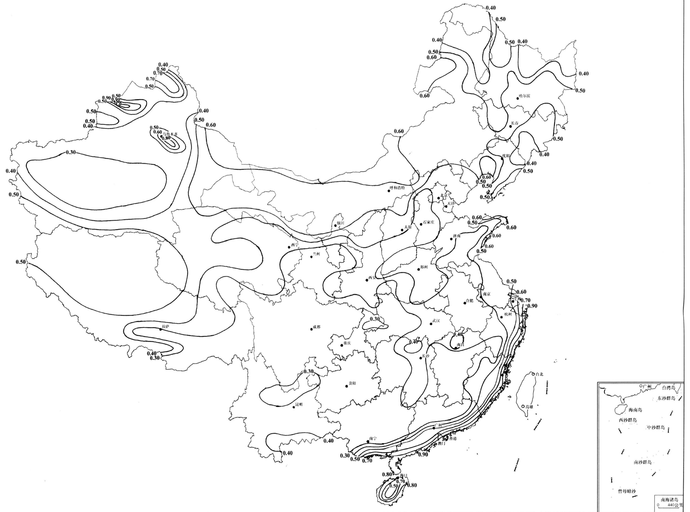
图 E. 6.3 全国基本风压分布图(kN/m²)
