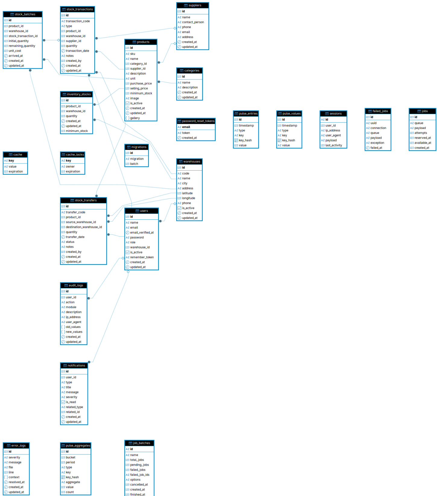
Gambar 6. ERD SmartStock Pro
