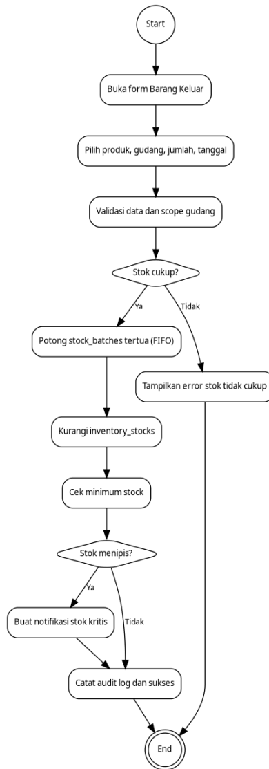
Gambar 3. Activity Diagram Barang Keluar
