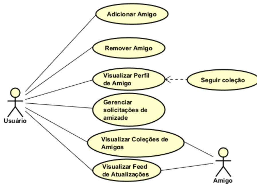
Figura 5 – Perfil e Social
