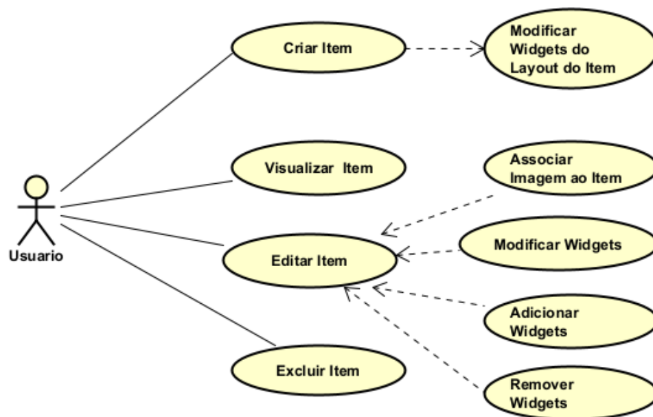
Figura 2 – Interações Com Itens da Coleção
