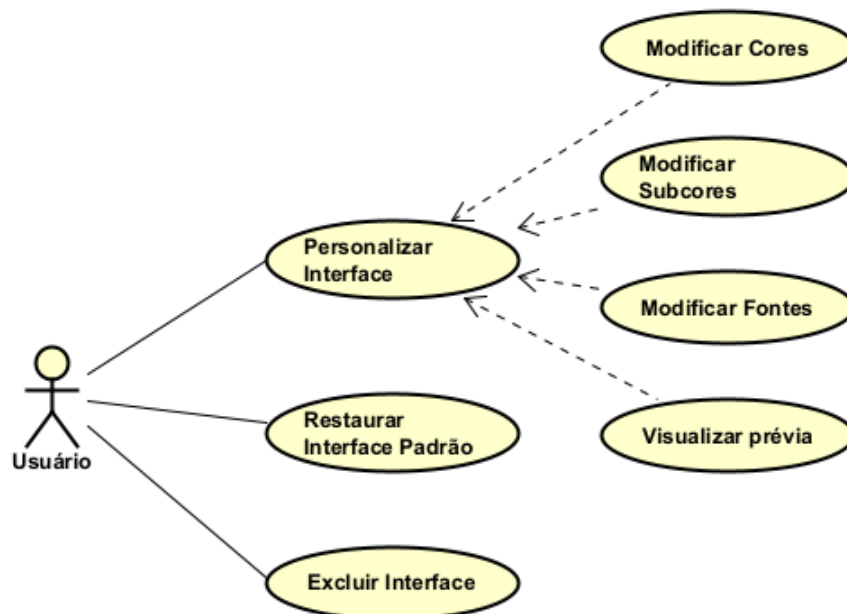
Figura 3 – Personalização da Plataforma
