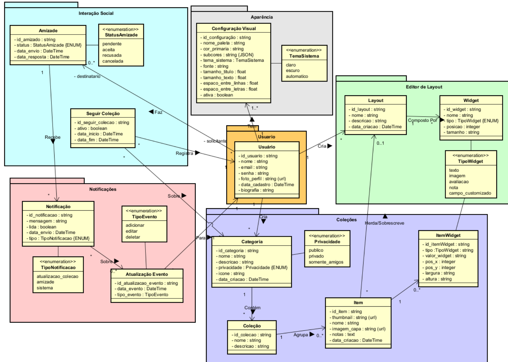
Figura 8 – Modelo de Domínio
