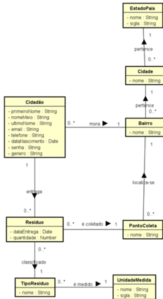
Figura 6 – Modelo de Domínio
