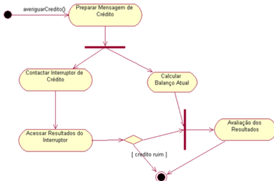
Figura 7 – Diagrama de Atividades
