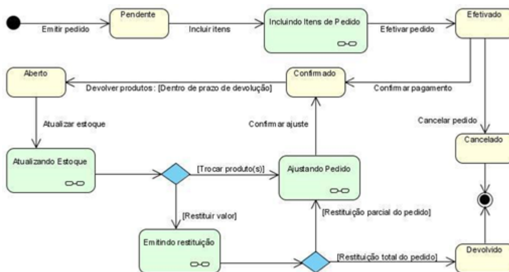
Figura 8 – Diagrama de Estados
