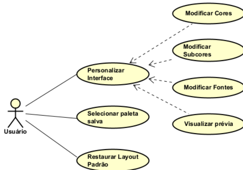
Figura 3 – Personalização da Plataforma
