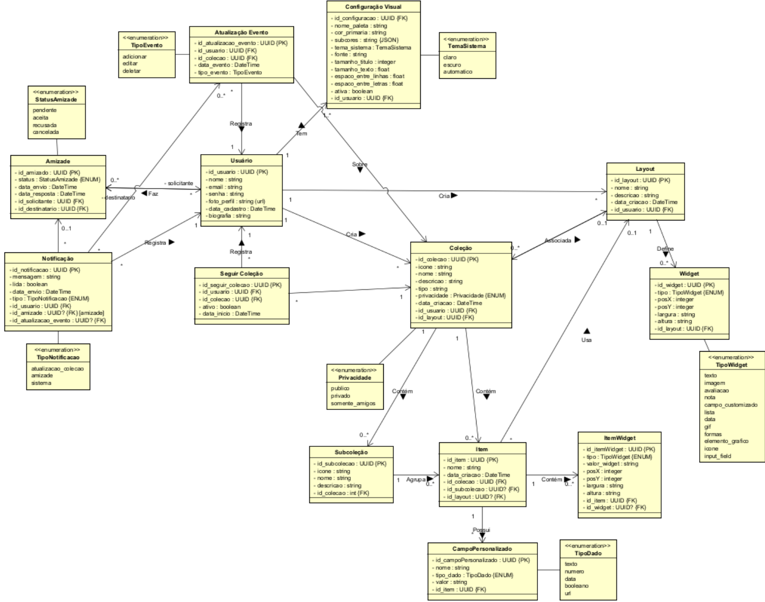
Figura 8 – Modelo de Domínio
