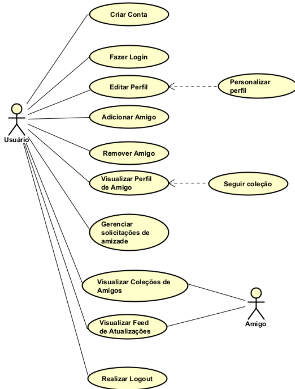
Figura 5 – Perfil e Social
